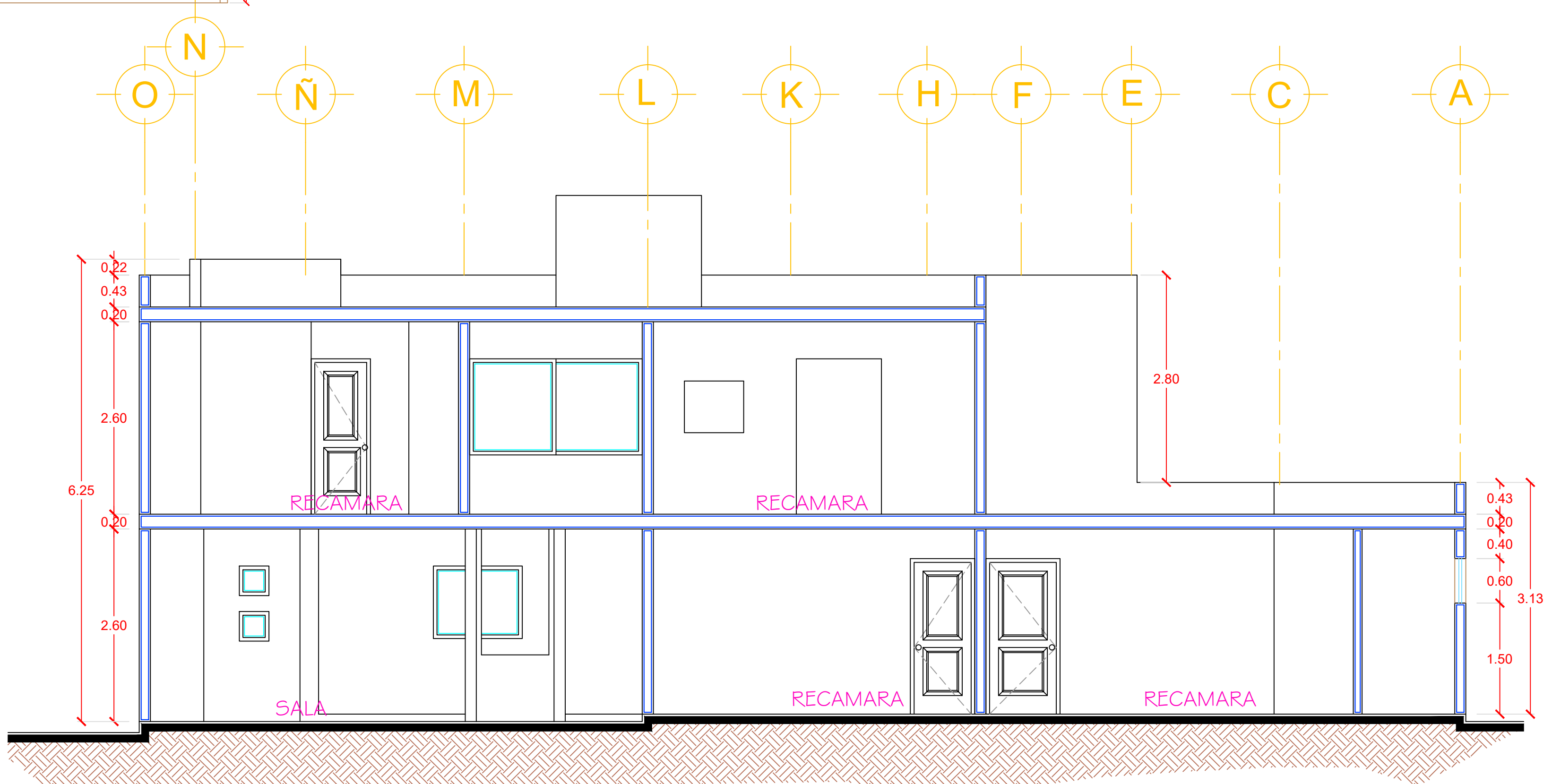
CORTE LONGITUDINAL A - A'
