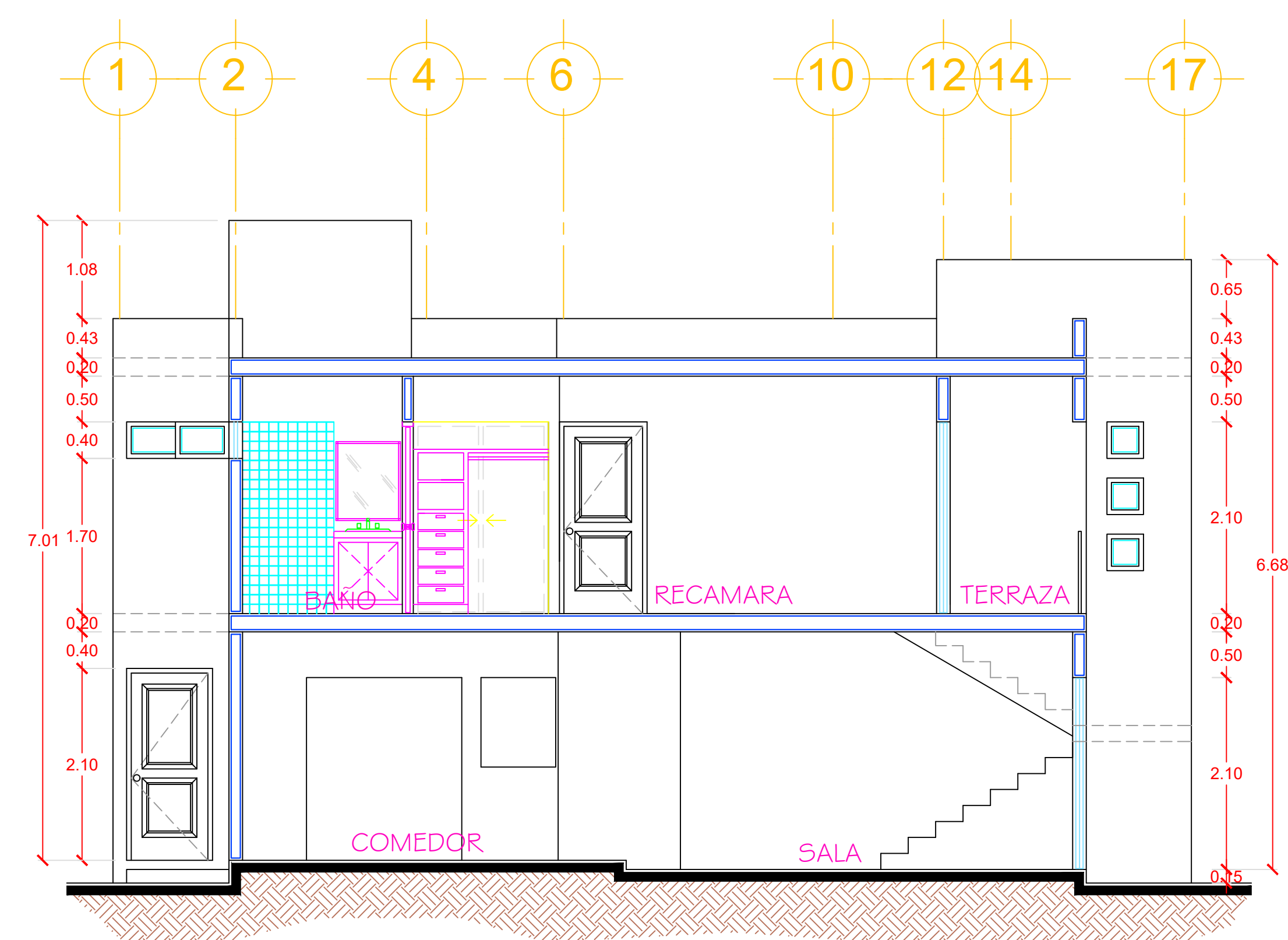
CORTE TRANSVERSAL B - B'
