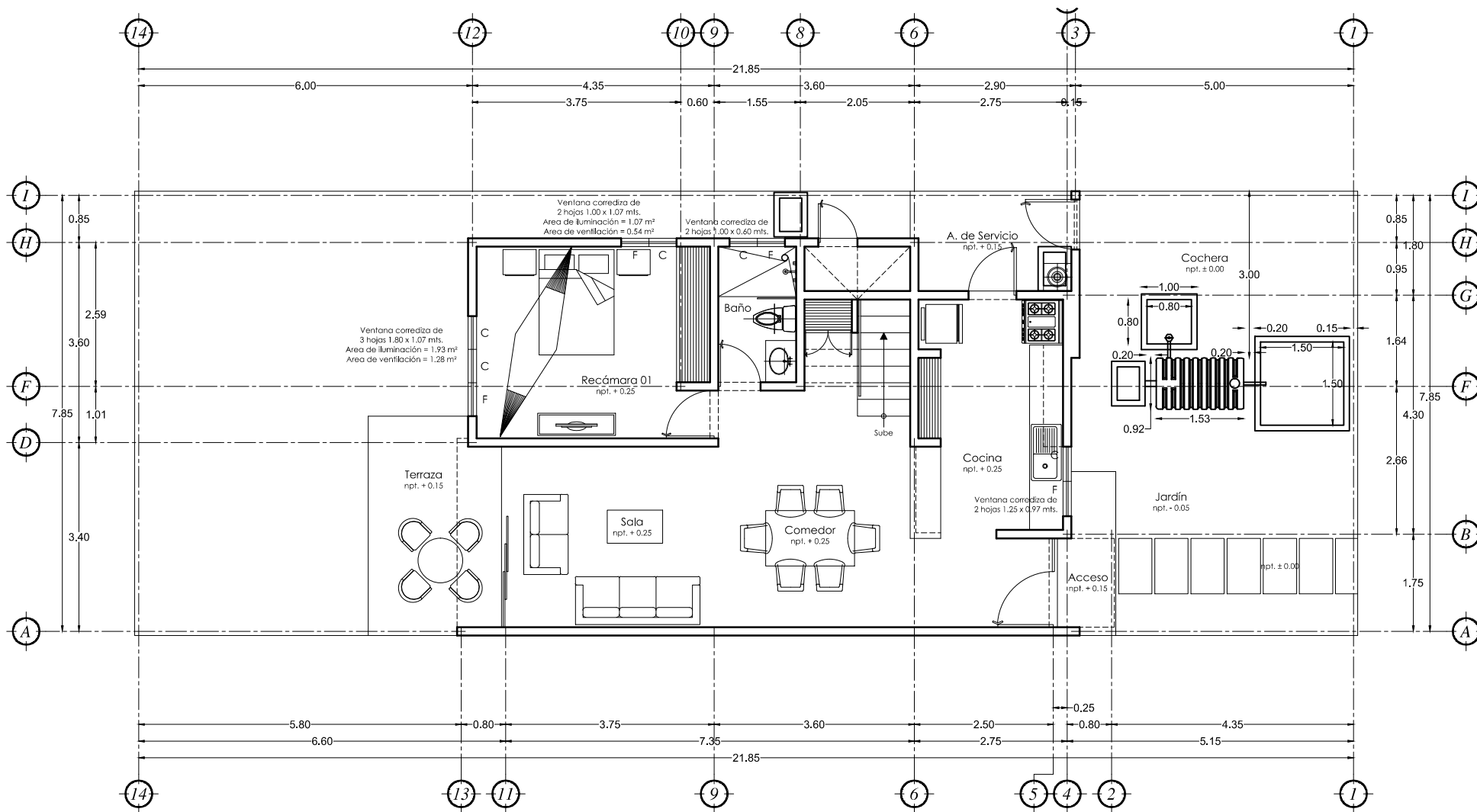
PLANTA BAJA
