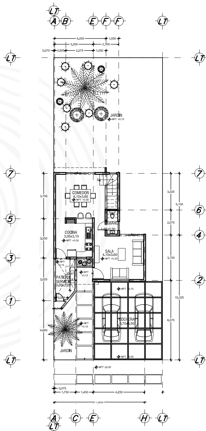
PLANTA BAJA AREA: 48.31M2
