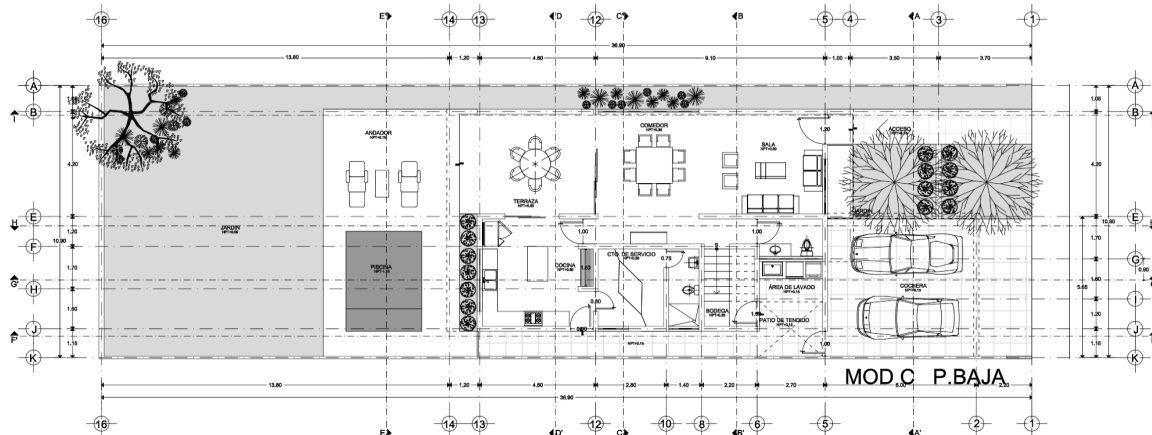
PLANTA BAJA ARQUITECTÓNICA
