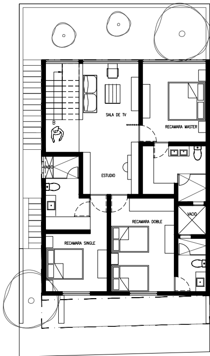
PLANTA ALTA
