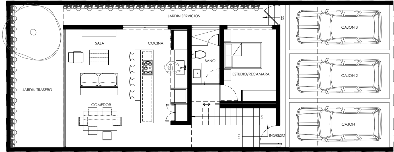
PLANTA BAJA
