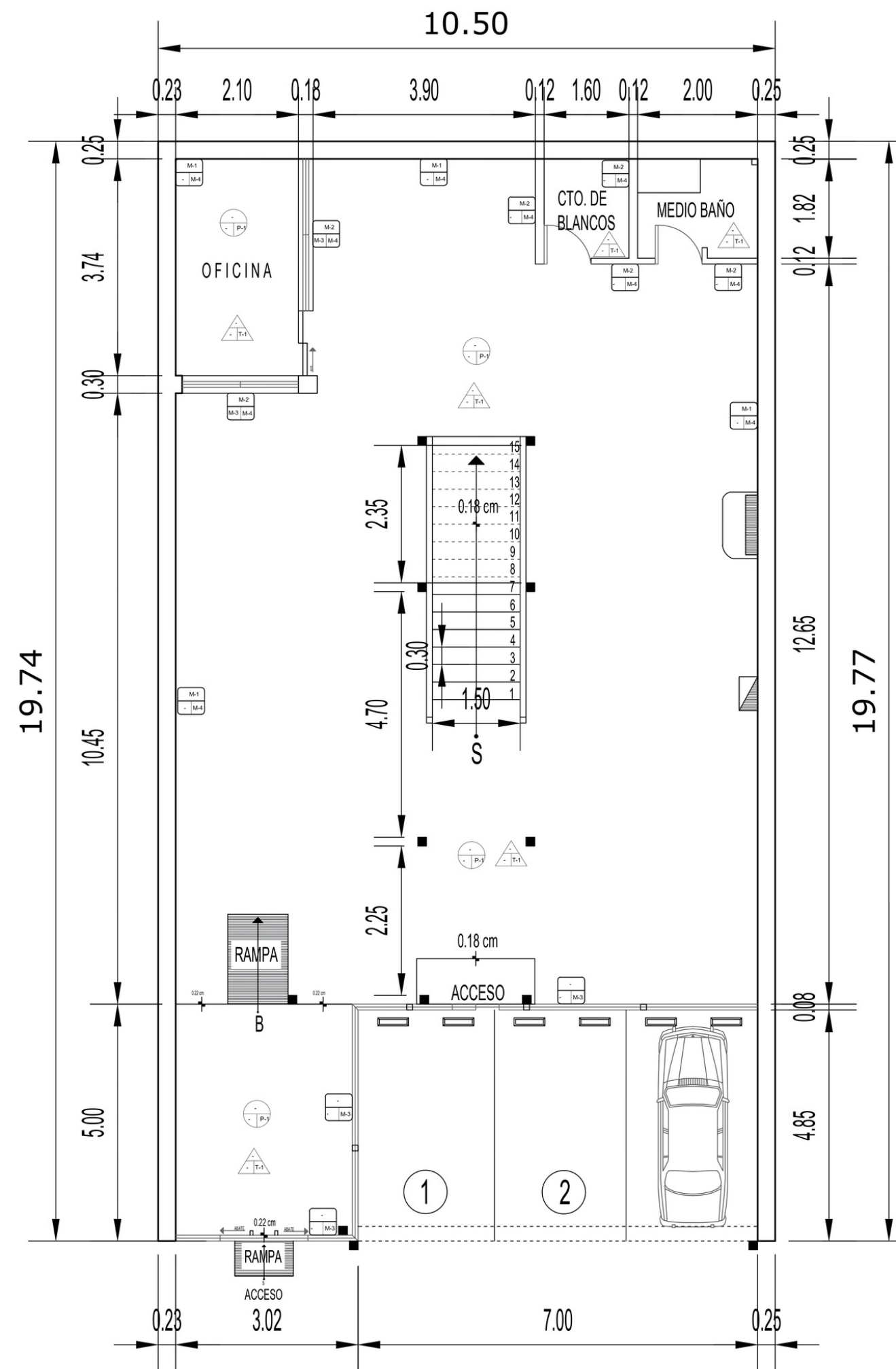
PLANTA BAJA
