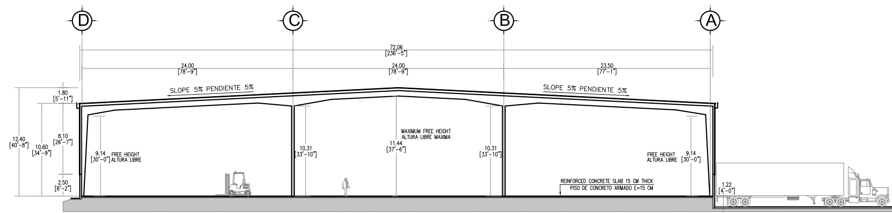
CROSS SECTION A - A' CORTE A - A'
