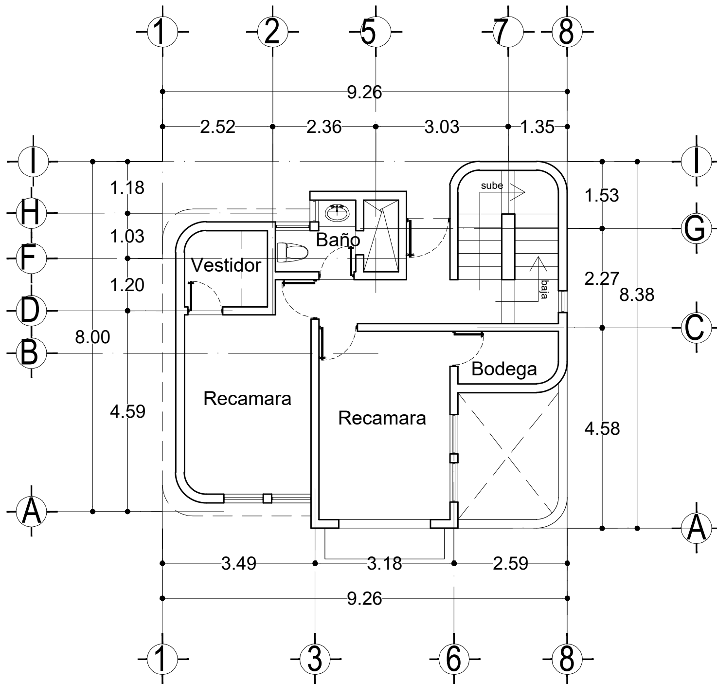
3ra Planta Arquitectónica
