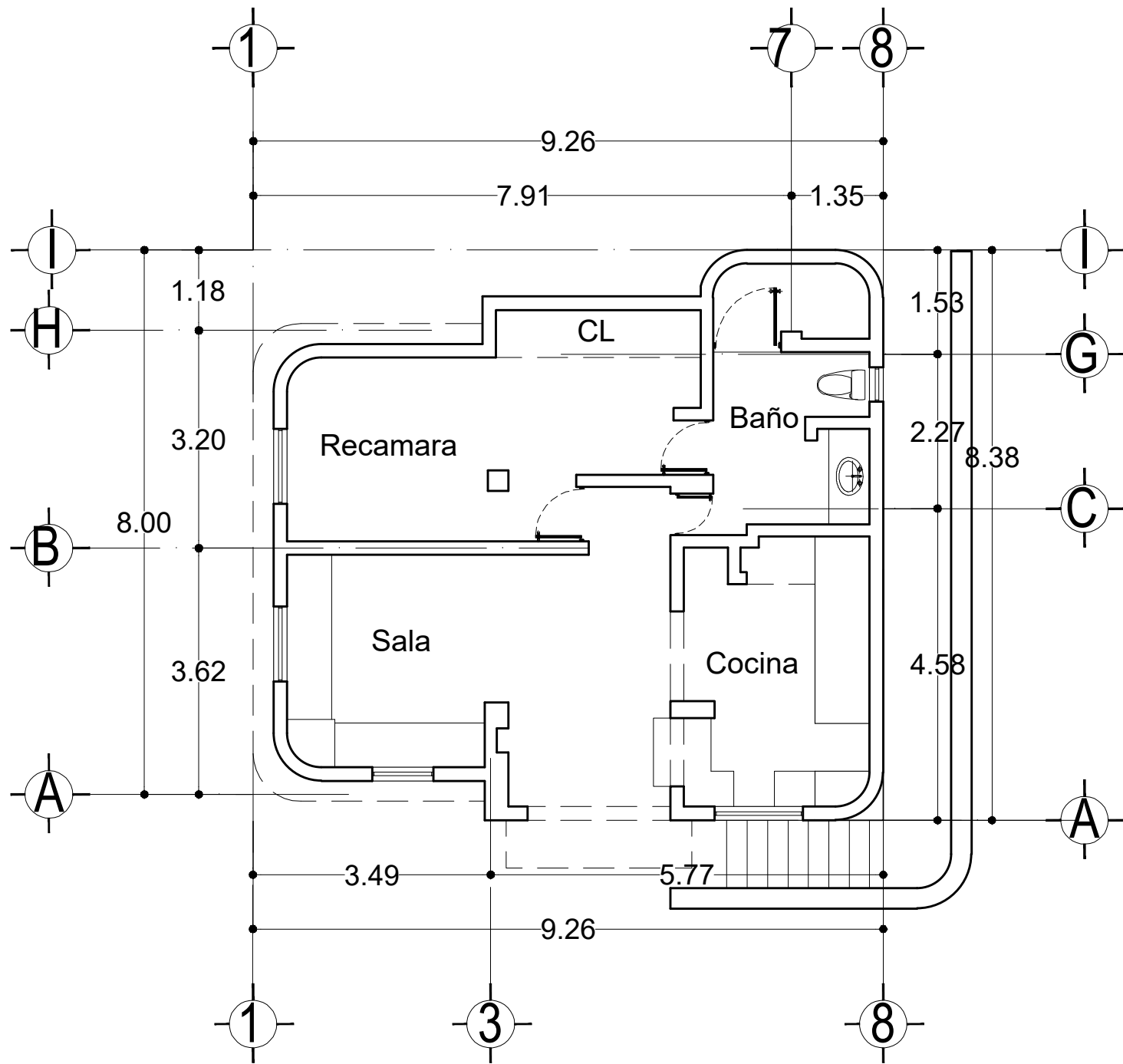
1ra Planta Arquitectónica
