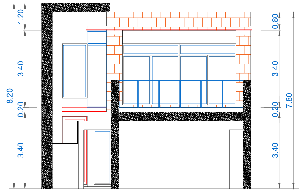
Elevacion Principal 1
