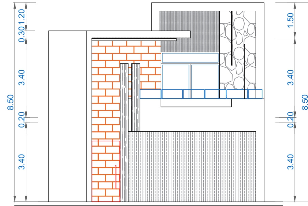
Elevacion Principal 2
