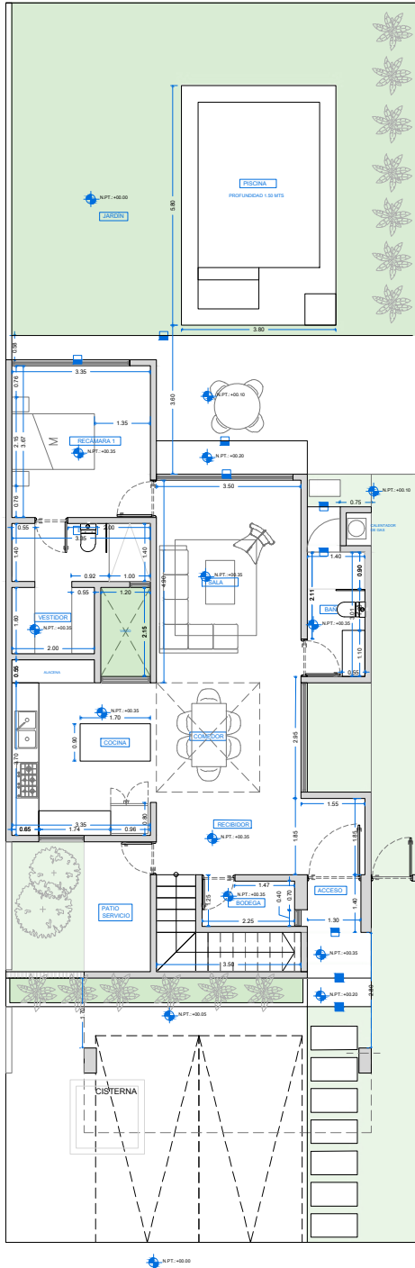
PLANTA BAJA
