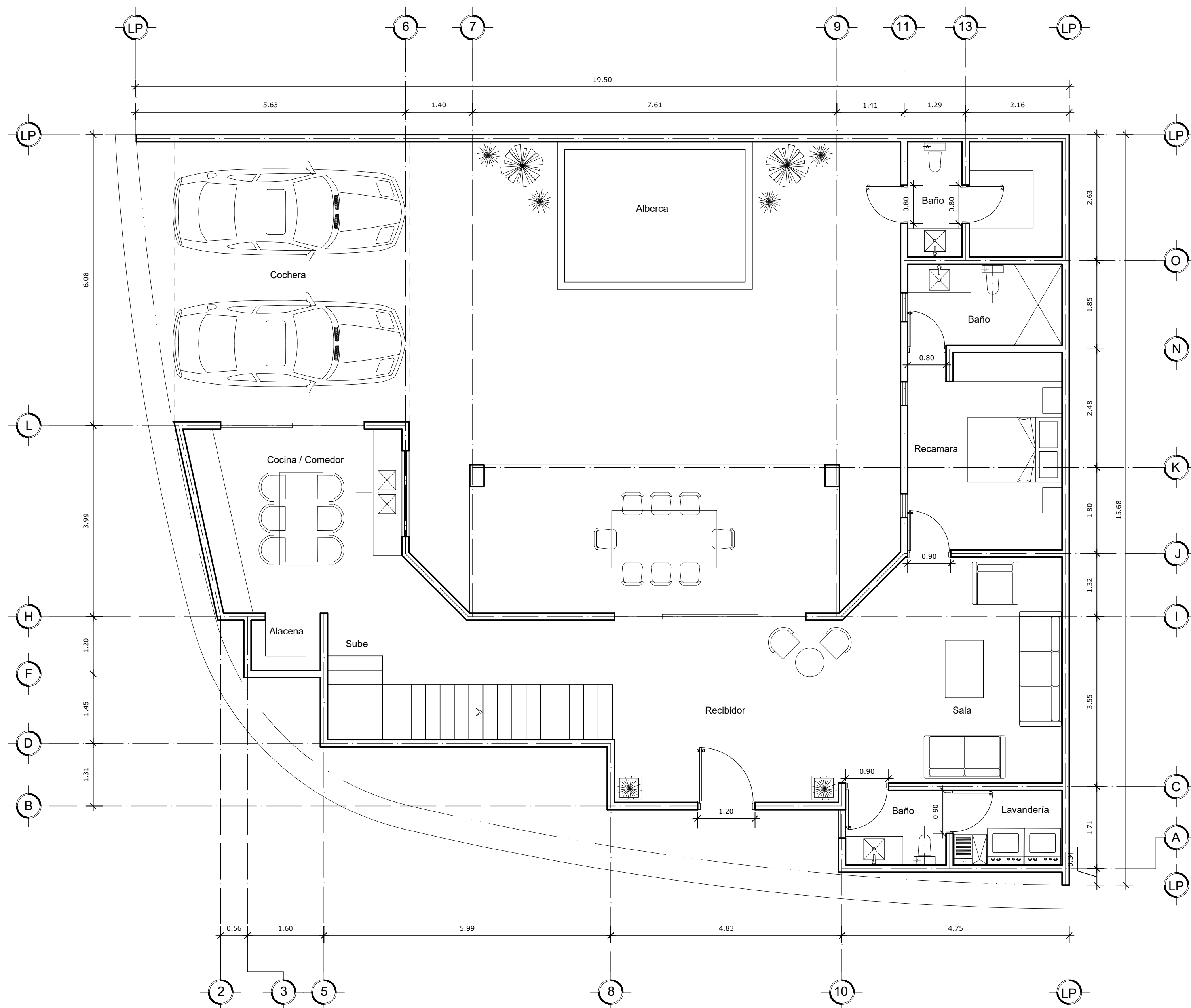
PLANTA BAJA 169.7 m2
