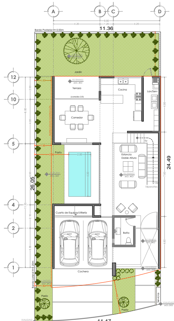
planta baja N+0.40 PASEO COUNTRY LT 159 PROYECTO ARQUITECTÓNICO
