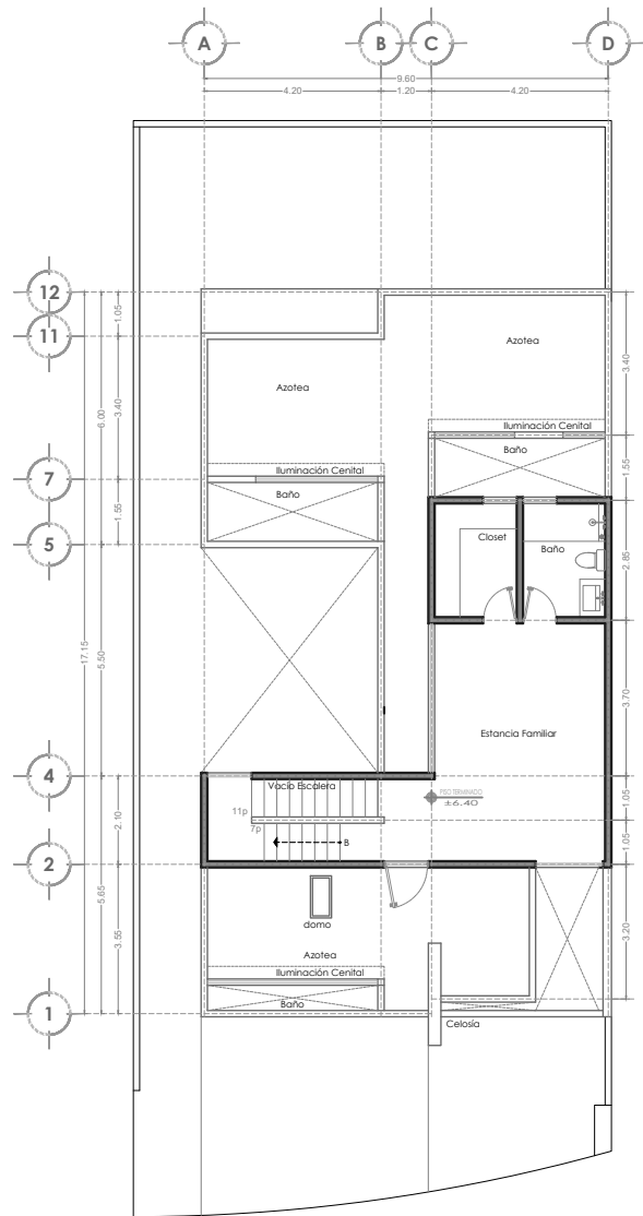
tercer nivel N+6.40 PASEO COUNTRY LT 159 PROYECTO ARQUITECTÓNICO
