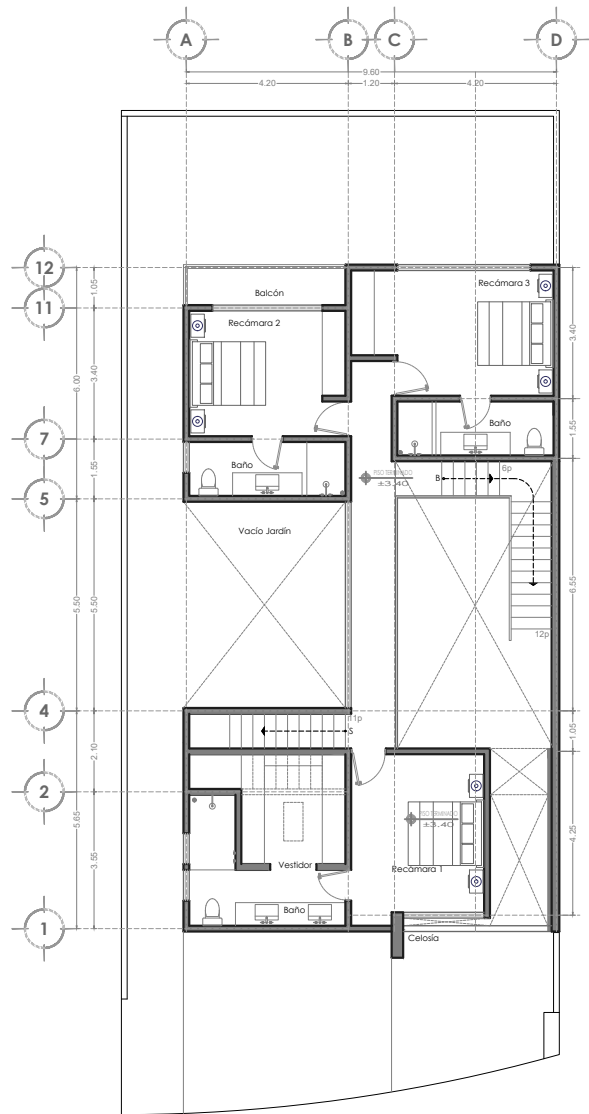
segundo nivel N+3.40 PASEO COUNTRY LT 159 PROYECTO ARQUITECTÓNICO
