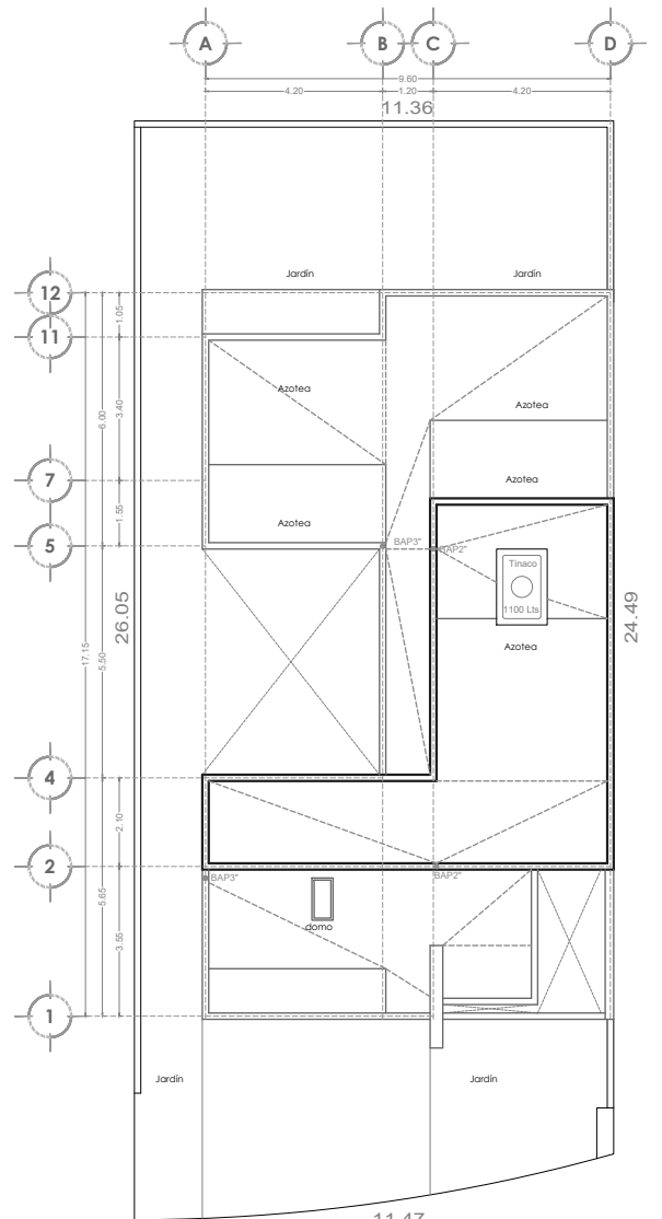
planta de azotea PASEO COUNTRY LT 159 PROYECTO ARQUITECTÓNICO
