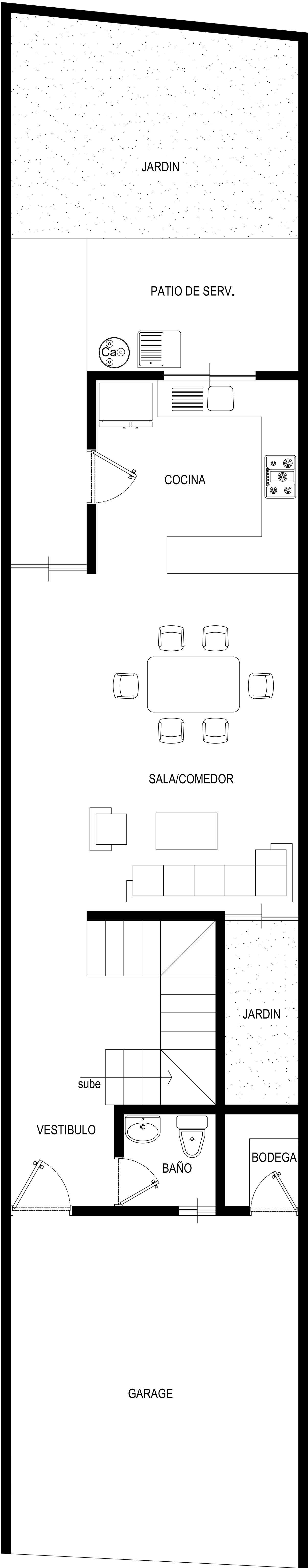
PLANTA BAJA SUP. CONST. 96.68M 2
