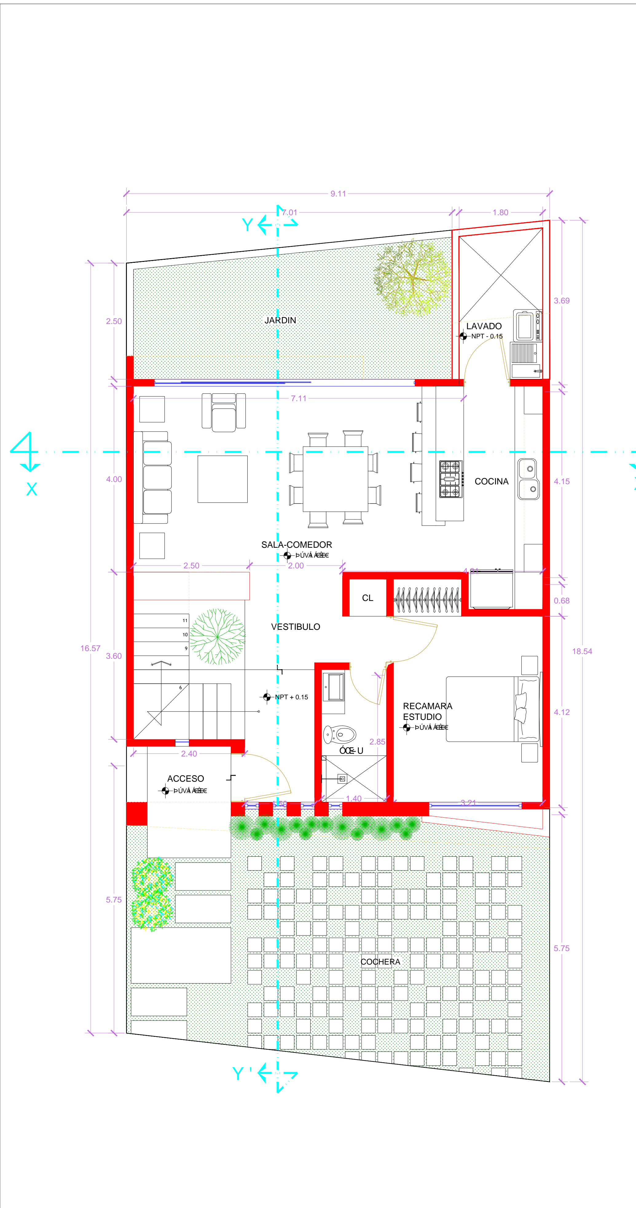
PLANTA BAJA 89.00 M2
