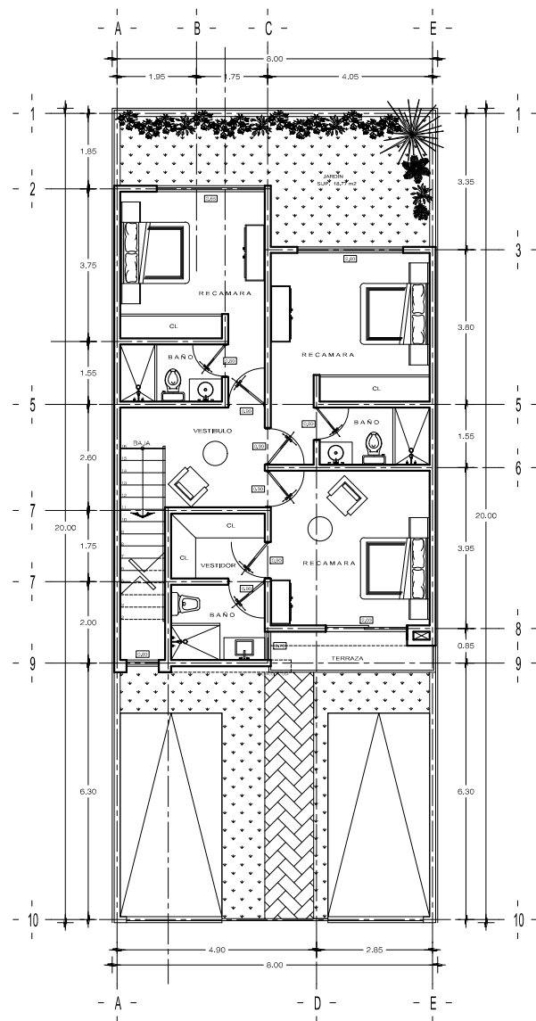
PLANTA ALTA 89.75 m 2
