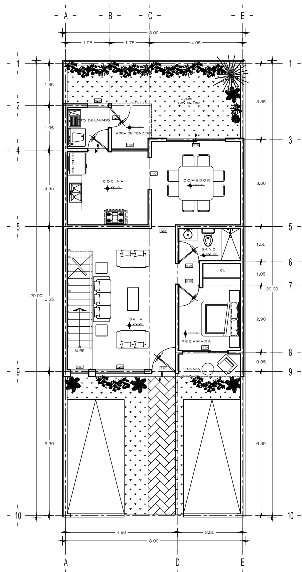
PLANTA BAJA 87.70 m 2
