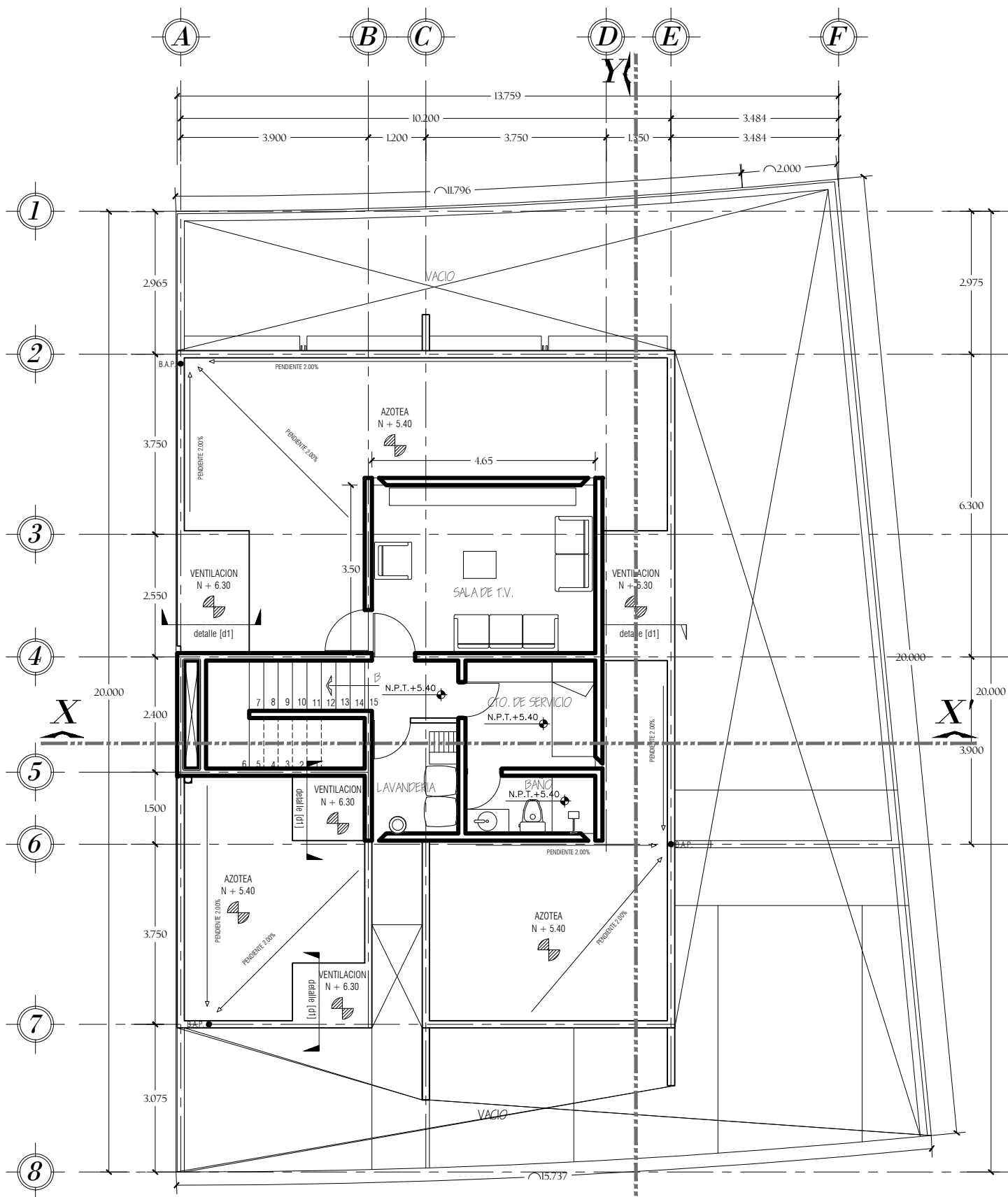
PLANTA SEGUNDO NIVEL
