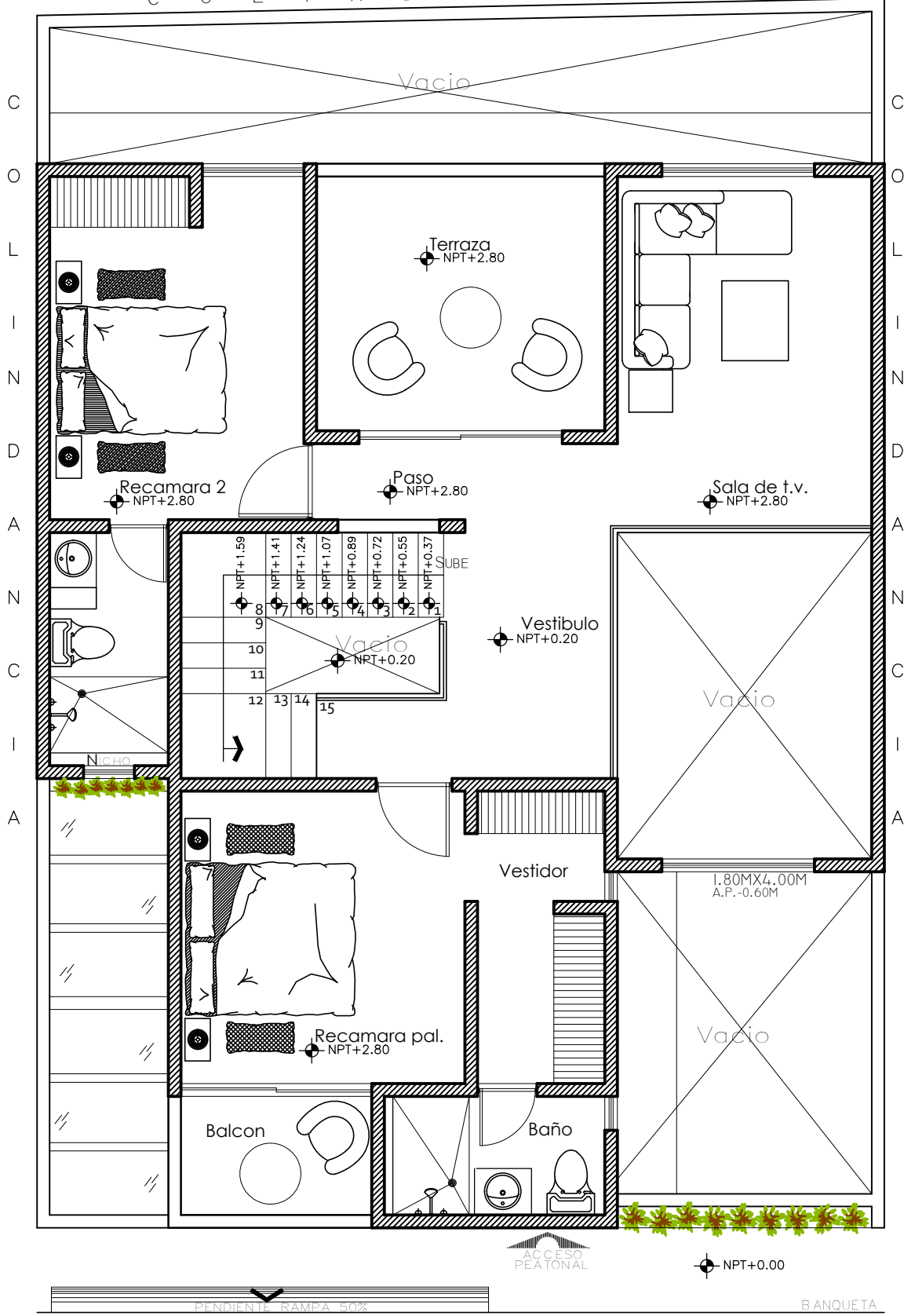
PLANTA ALTA Sup.89.63m 2 propuesta 5
