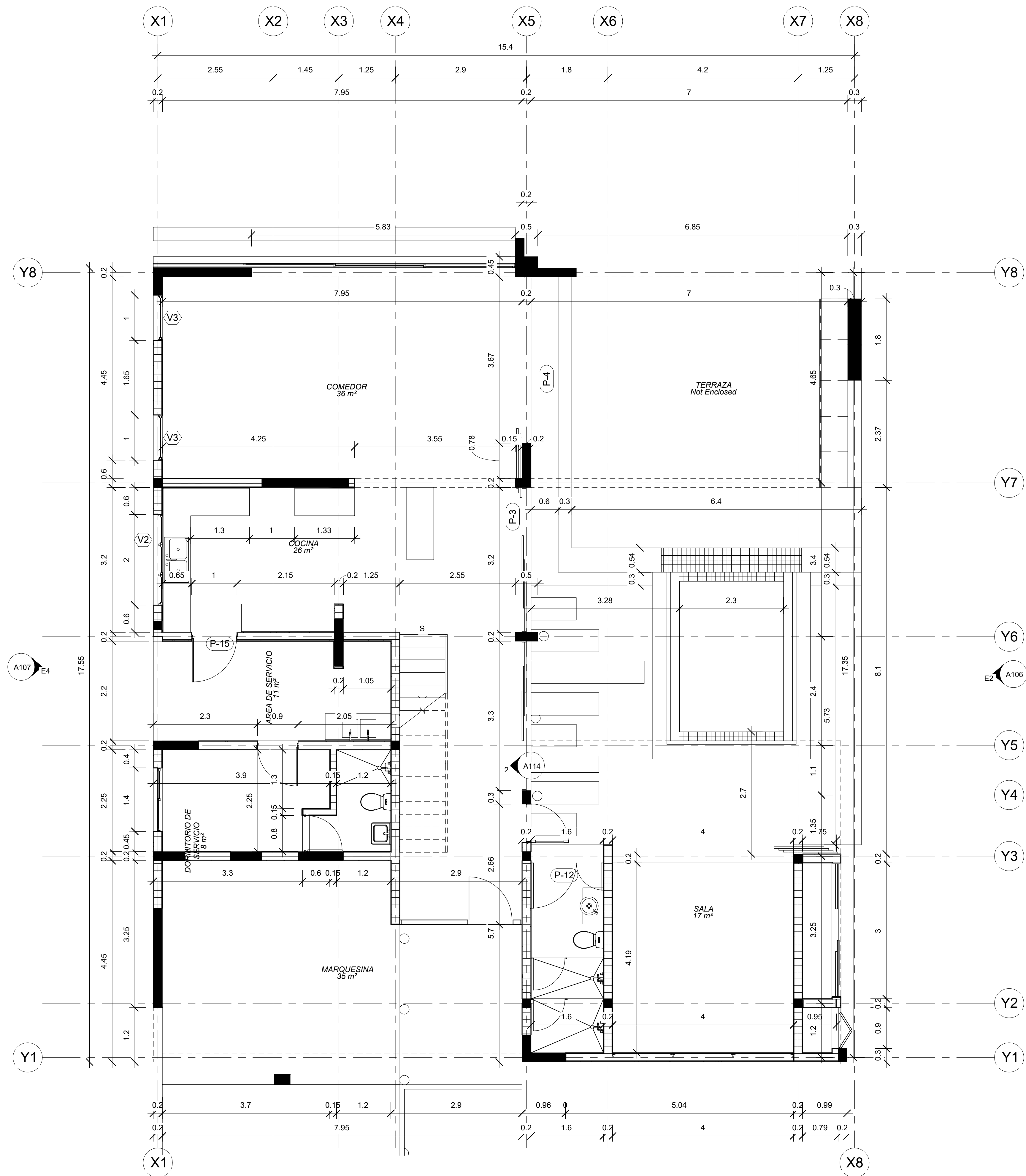
● Planta Dimensionada 1 Nivel 1 : 50
