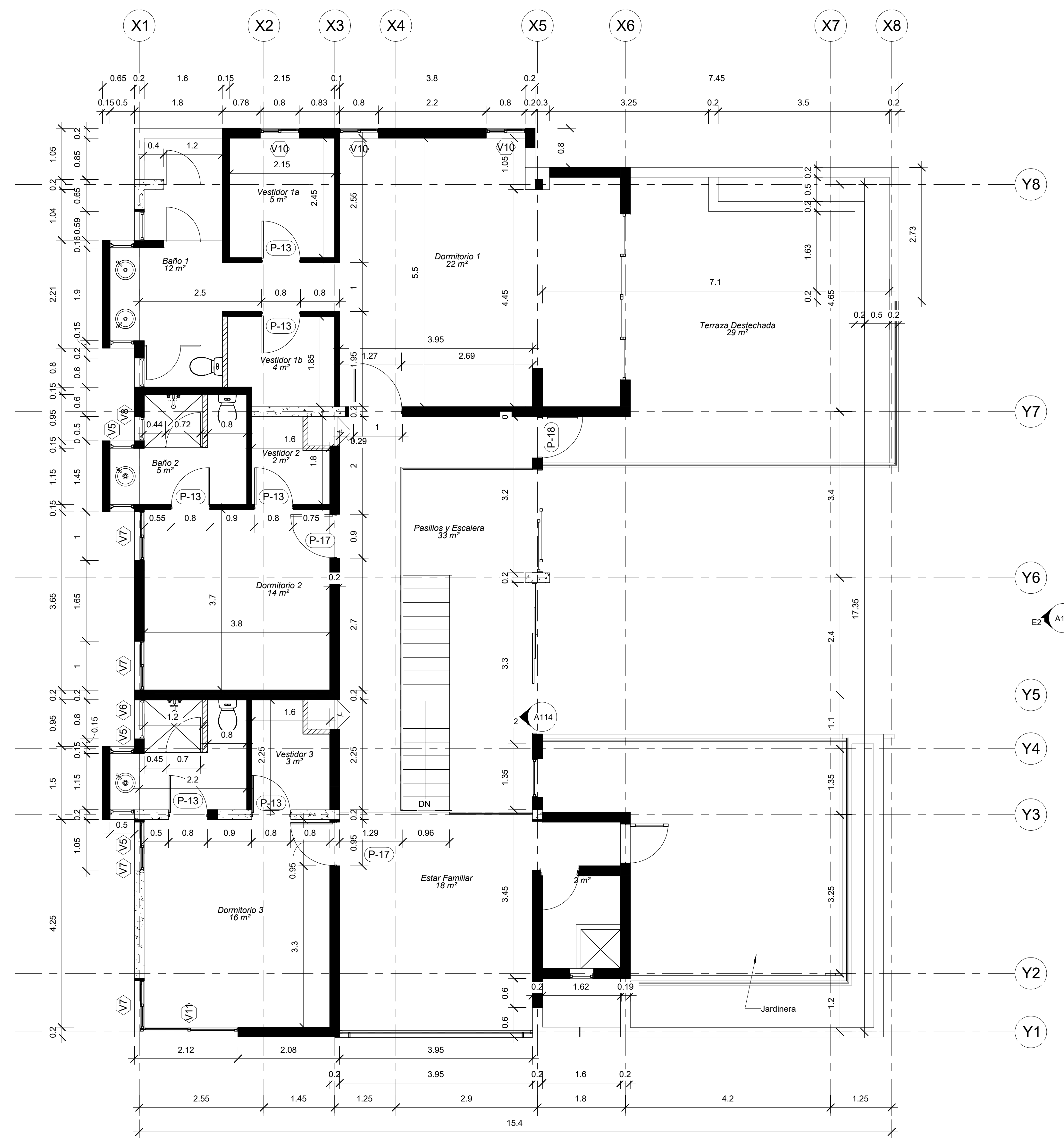
● Planta Dimensionada 2Nivel 1 : 50
