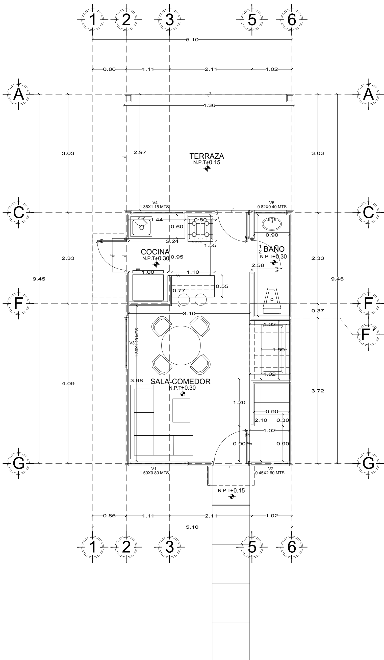
PLANTA ARQUITECTONICA PLANTA BAJA
