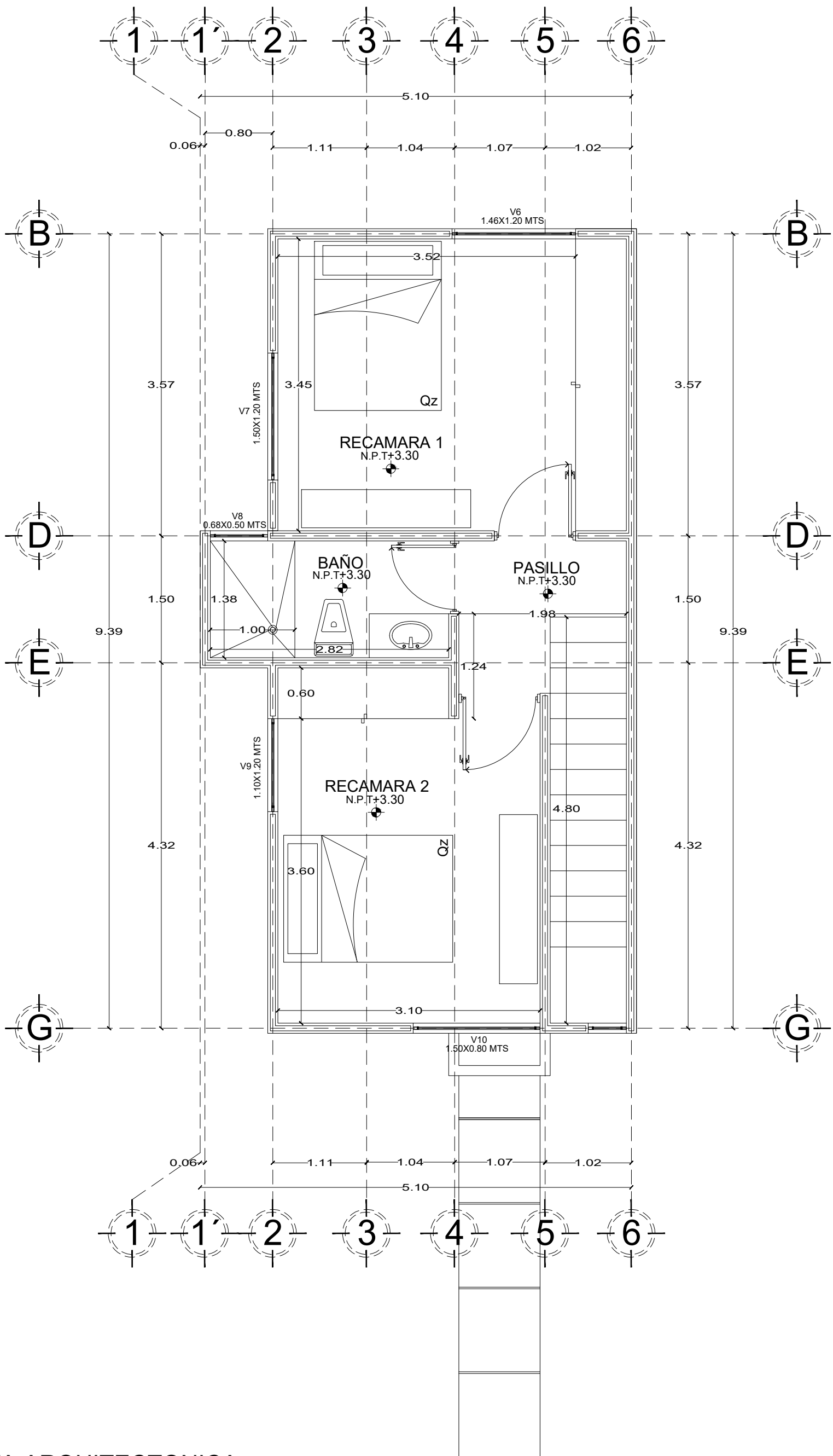
PLANTA ARQUITECTONICA PLANTA ALTA
