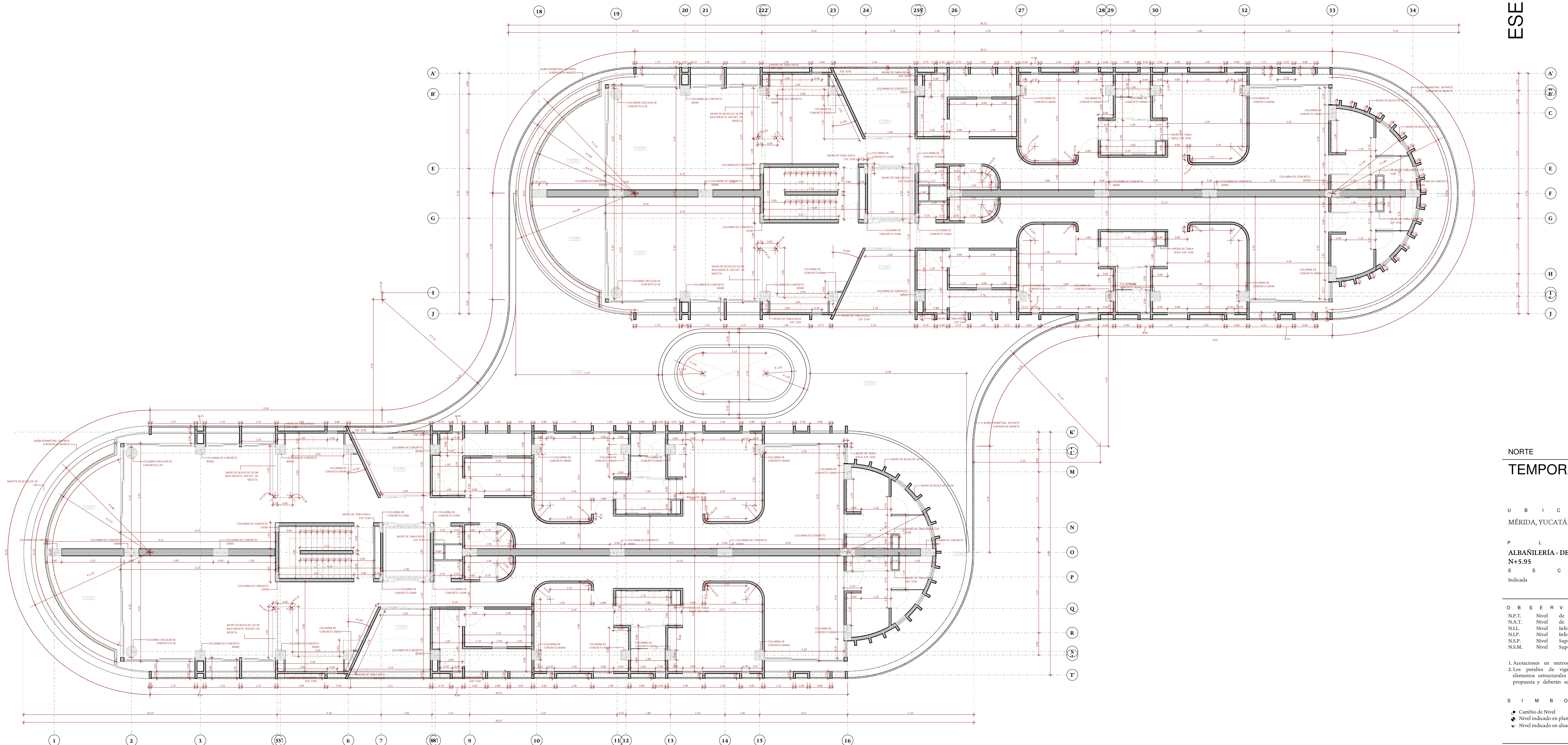
1 | ALB - N+5.95 - DEPTO CLÁSICO ESC 1 : 75
