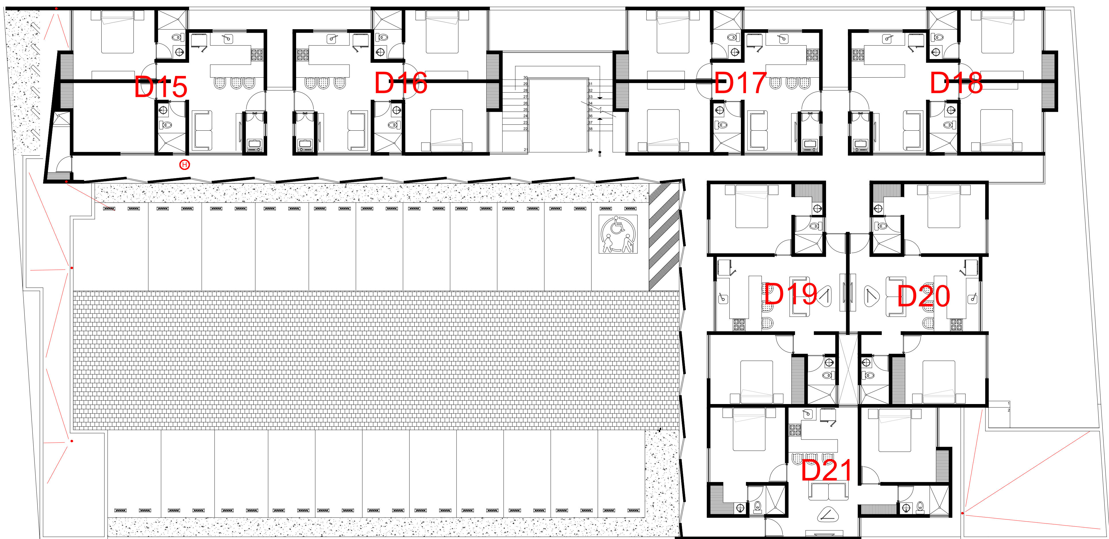
PLANTA SEGUNDO NIVEL
