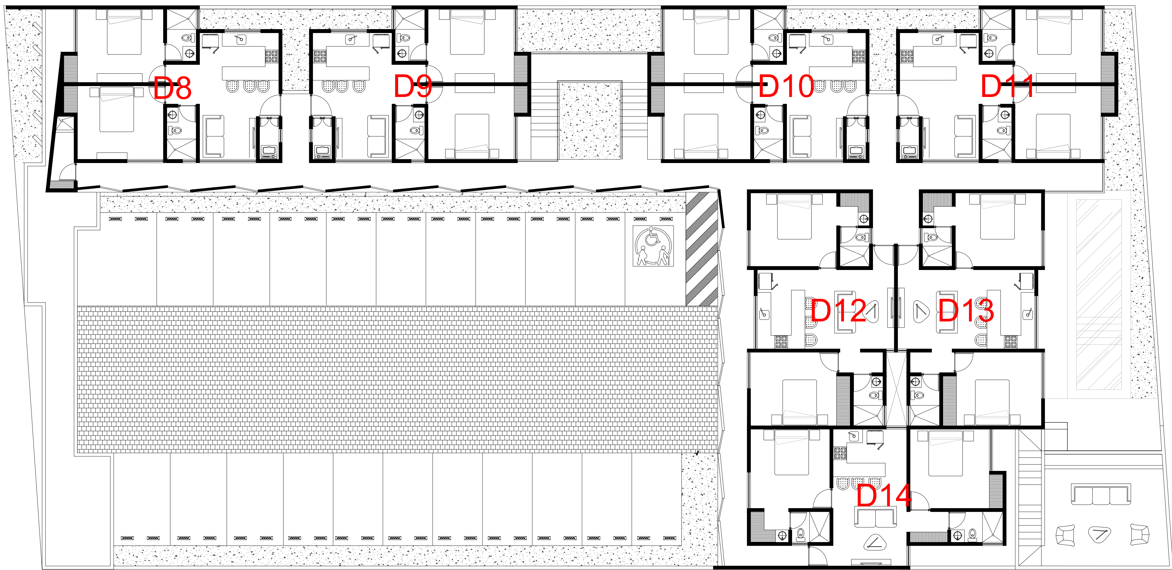
PLANTA PRIMER NIVEL
