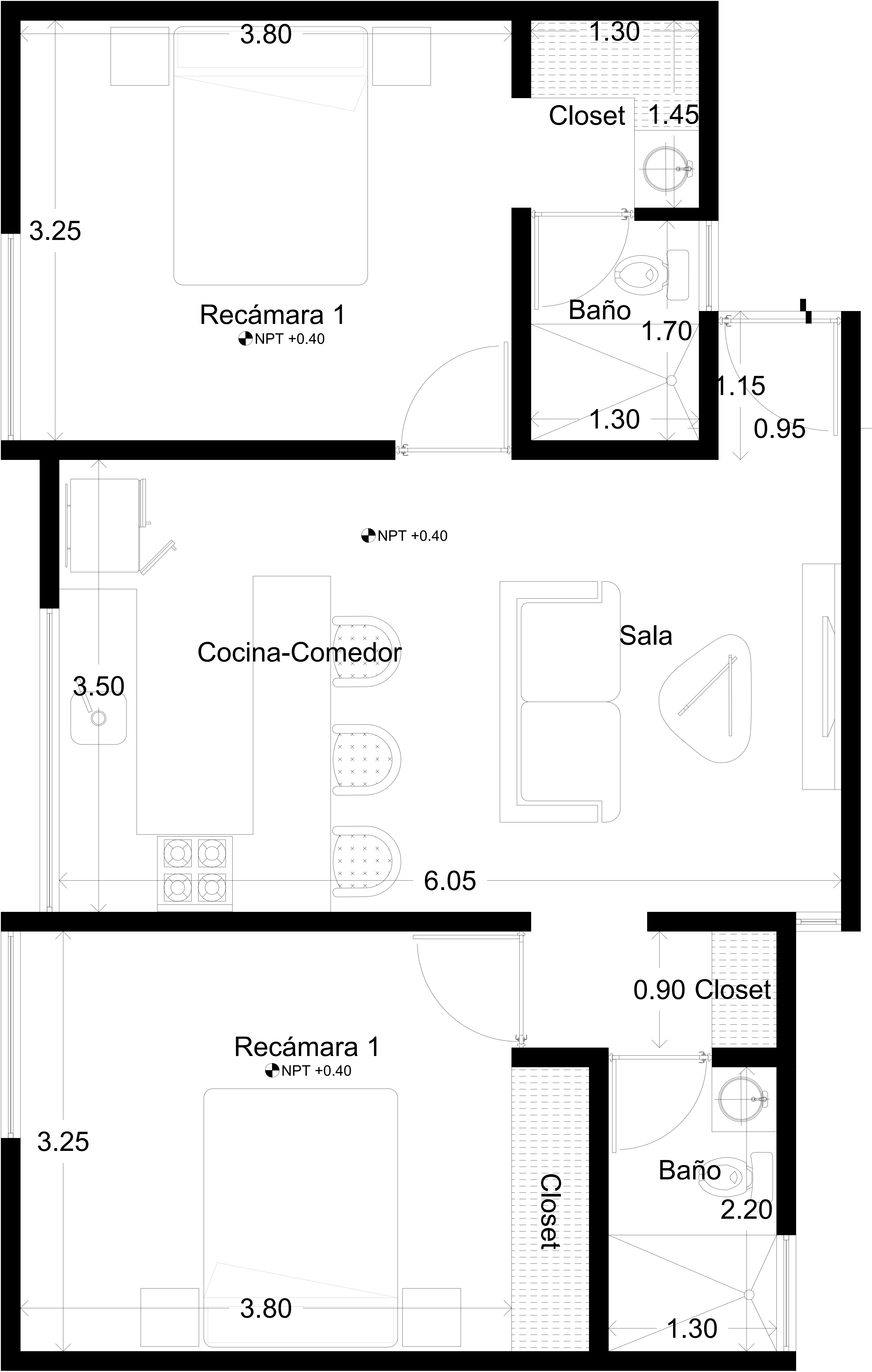
Planta Arquitectónica. Metros cuadrados:64.74 m2
