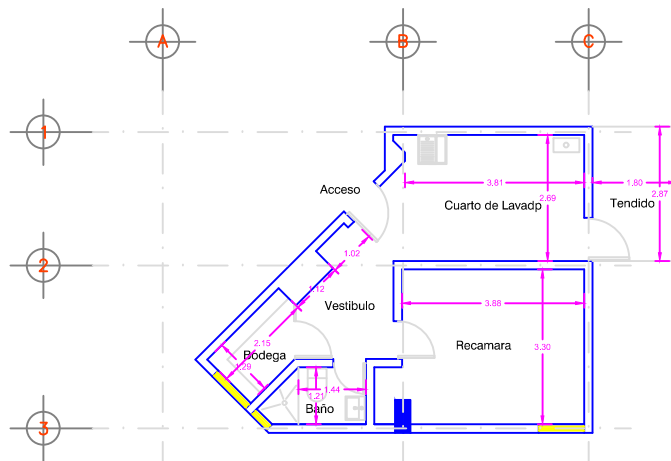
PLANTA DE SERVICIO PH-2 Carlos Dickens # 52 PH-2
