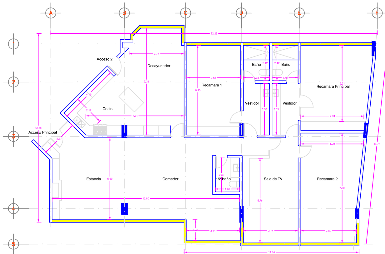
PLANTA ARQUITECTONICA Carlos Dickens # 52 PH-2
