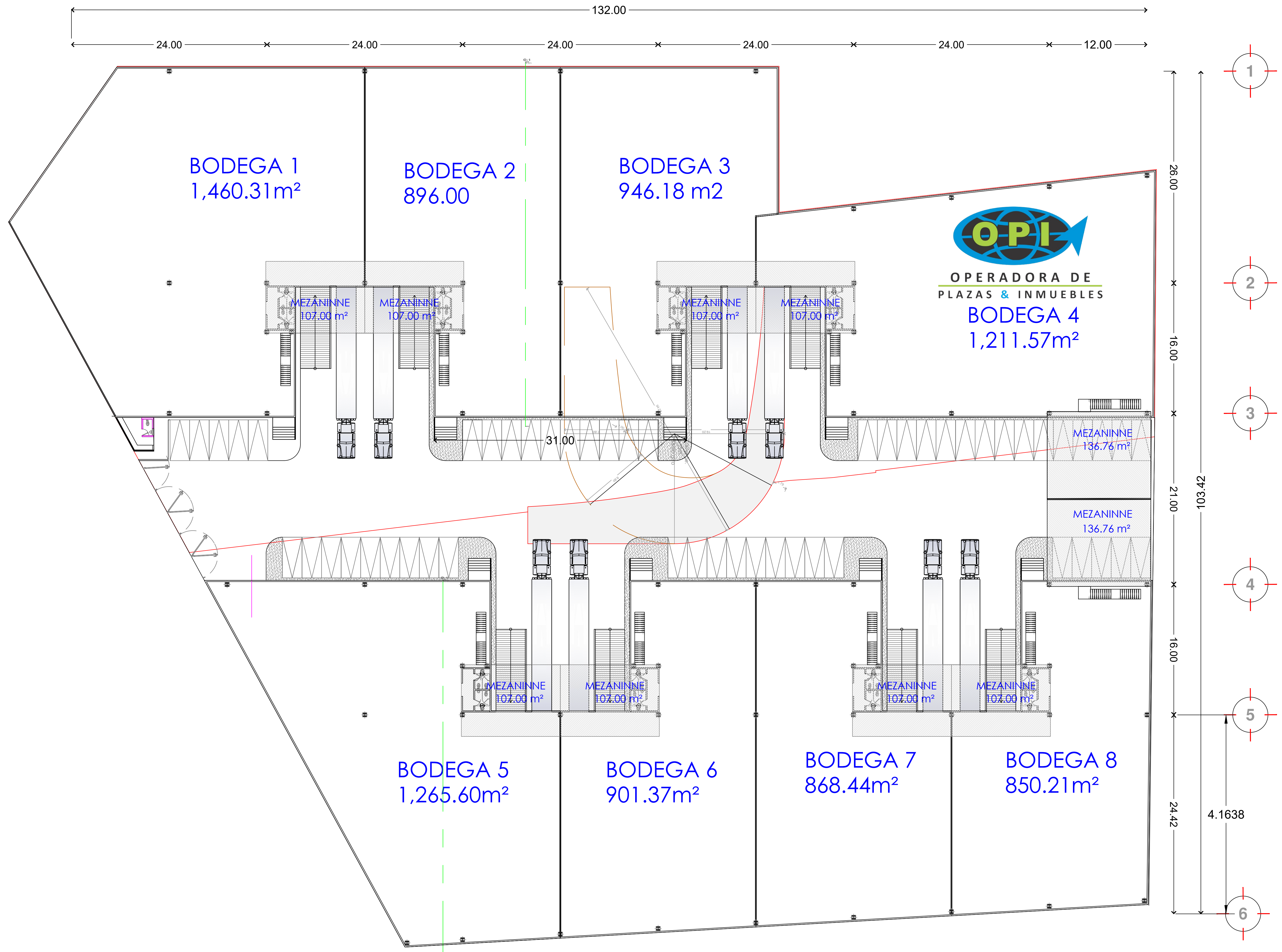
Planta General Arquitectonico. Acot. en metros Escala 1:500
