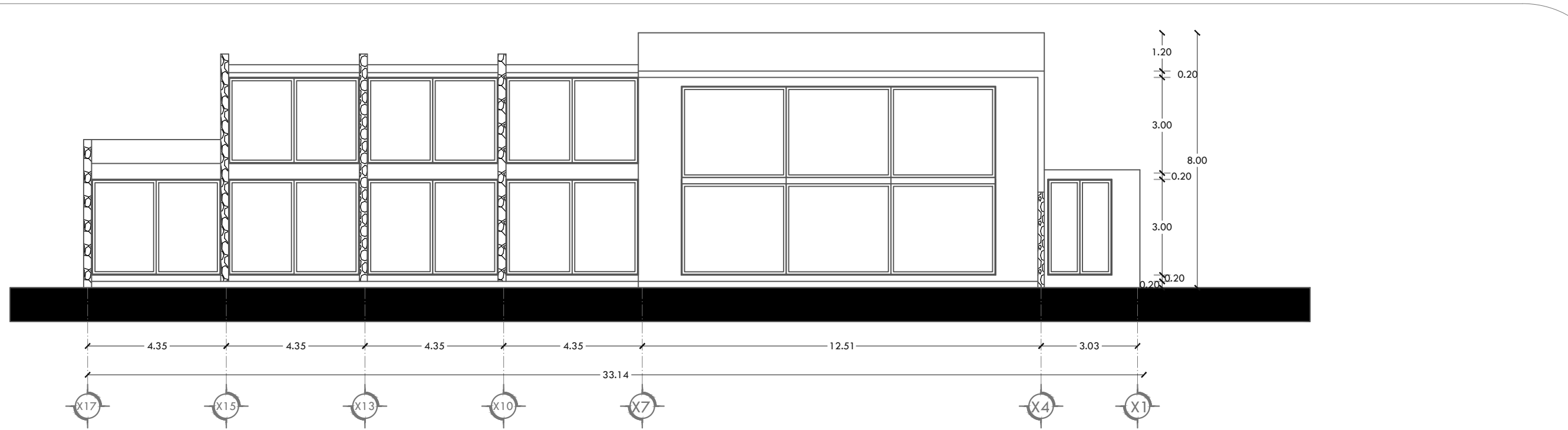
VISTA -3 Proyecto CASA SELVA 4 Nivel: 0 | Esc. S/E | Esc.G.
