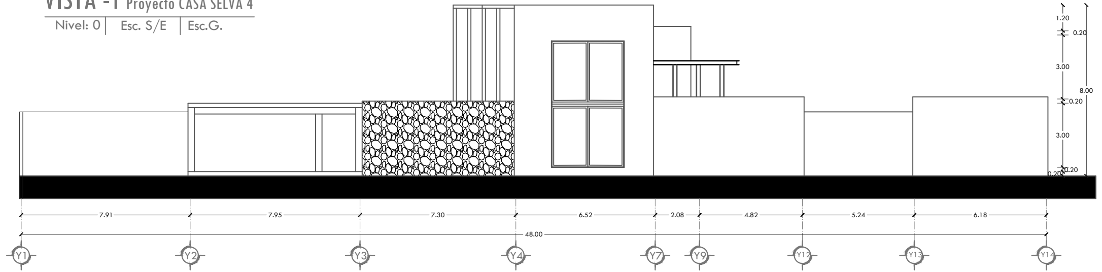
VISTA -2 Proyecto CASA SELVA 4 Nivel: 0 | Esc. S/E | Esc.G.
