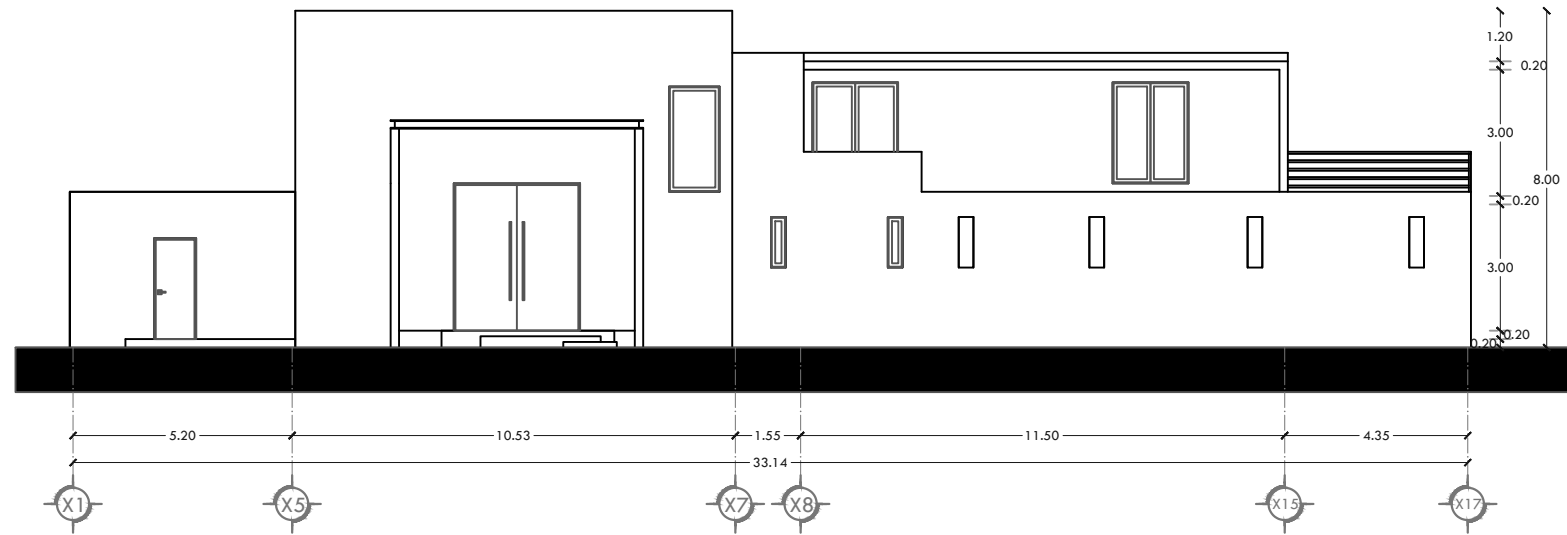
VISTA -1 Proyecto CASA SELVA 4 Nivel: 0 | Esc. S/E | Esc.G.
