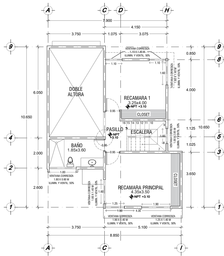
PLANTA ALTA ESC. 1:150
