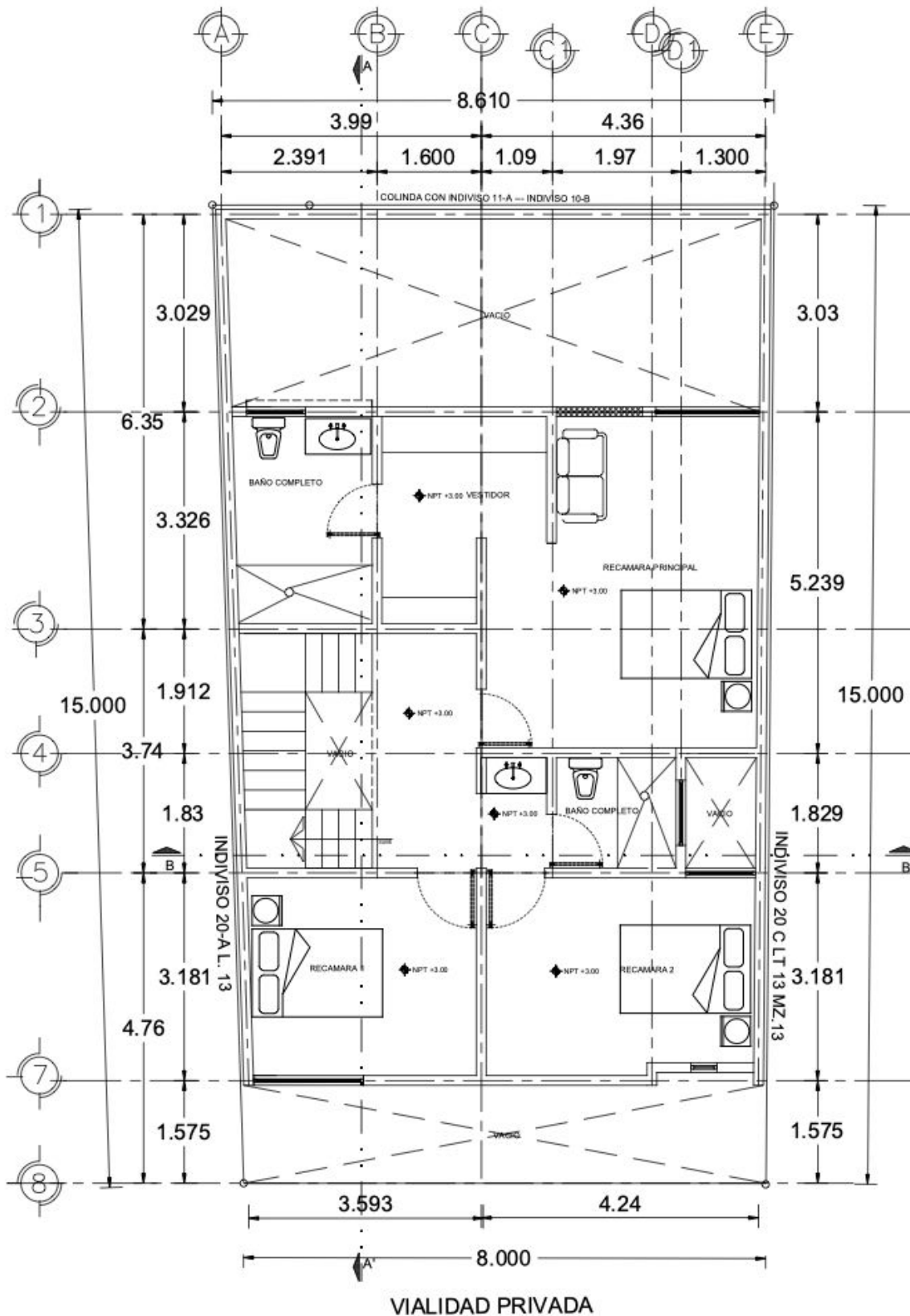
PLANTA ALTA 82.57 M2
