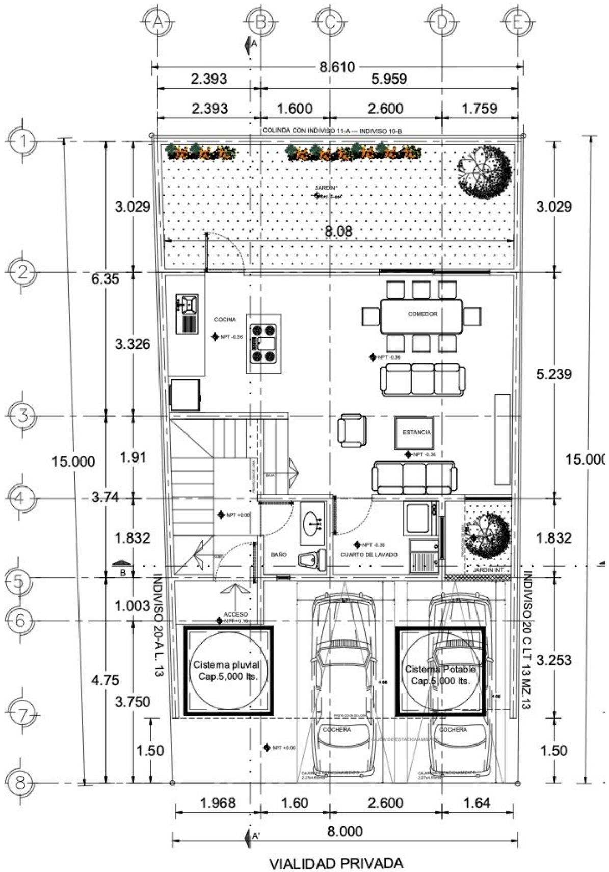
PLANTA BAJA 82.57 M2
