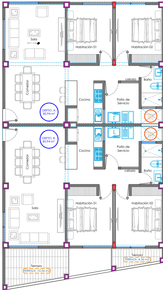
05 ARQUITECTÓNICO- PRIMER NIVEL TORRE LEXUS Departamento Tipo A 87.60 m 2 Departamento Tipo B 107.55 m 2
