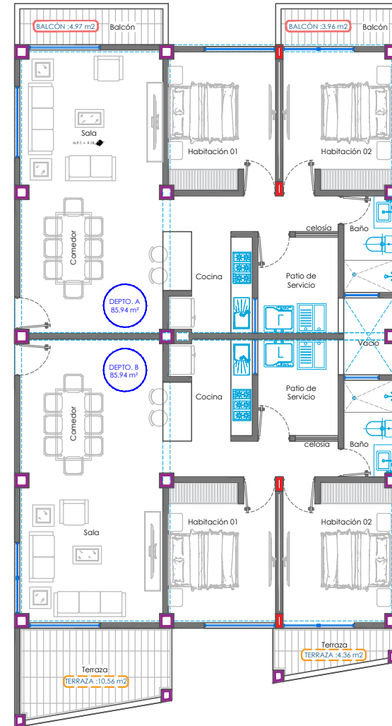
06 ARQUITECTÓNICO - 2° A 5° NIVEL TORRE LEXUS Departamento Tipo A 94.87 m 2 Departamento Tipo B 100.86 m 2
