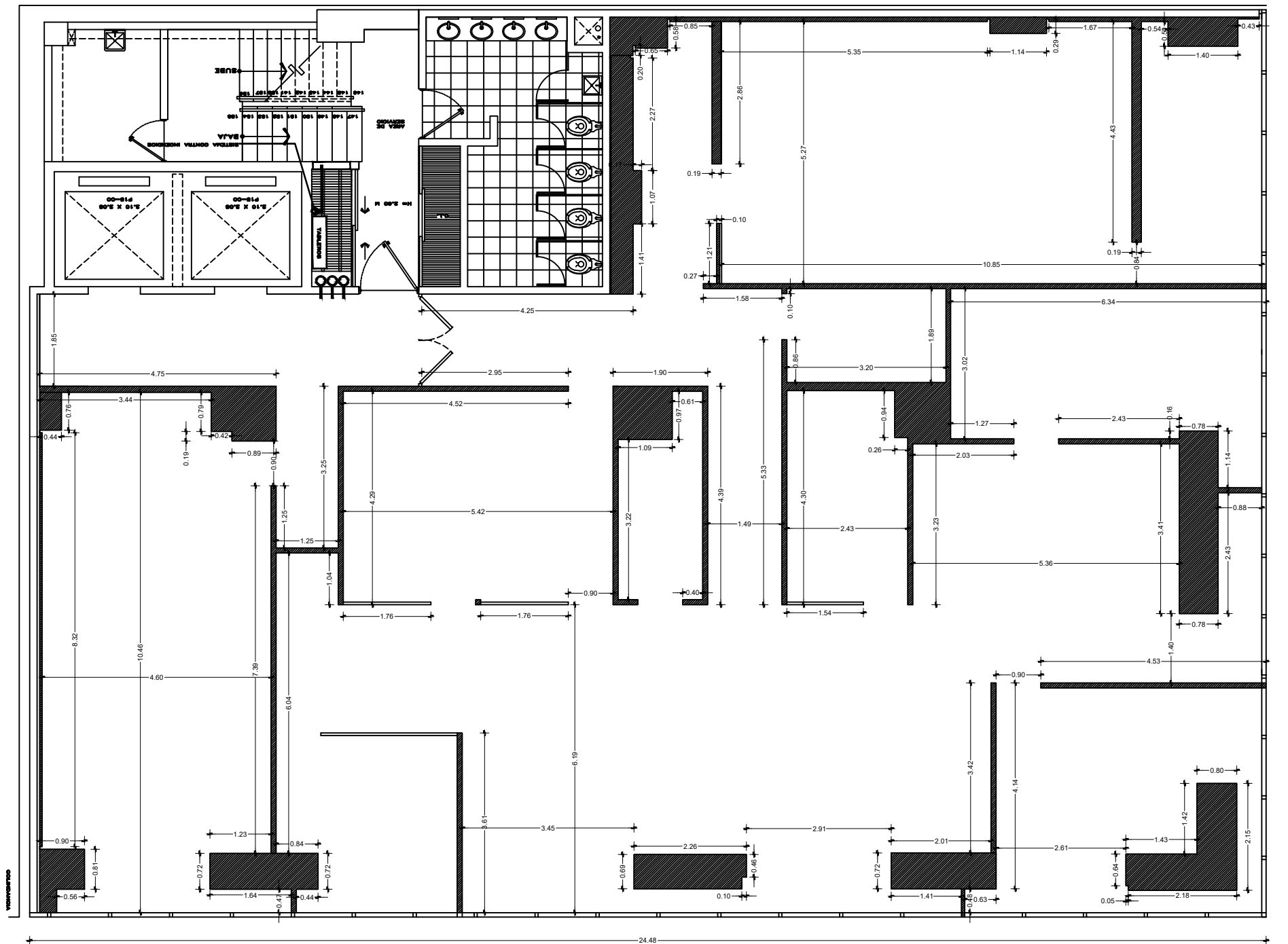
PLANTA CUARTO NIVEL (OFICINAS)
