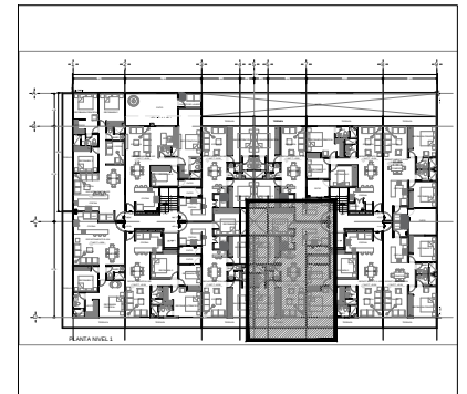
UBICACIÓN EN PLANTA NIVEL 2 DEPARTAMENTO "A-206"
