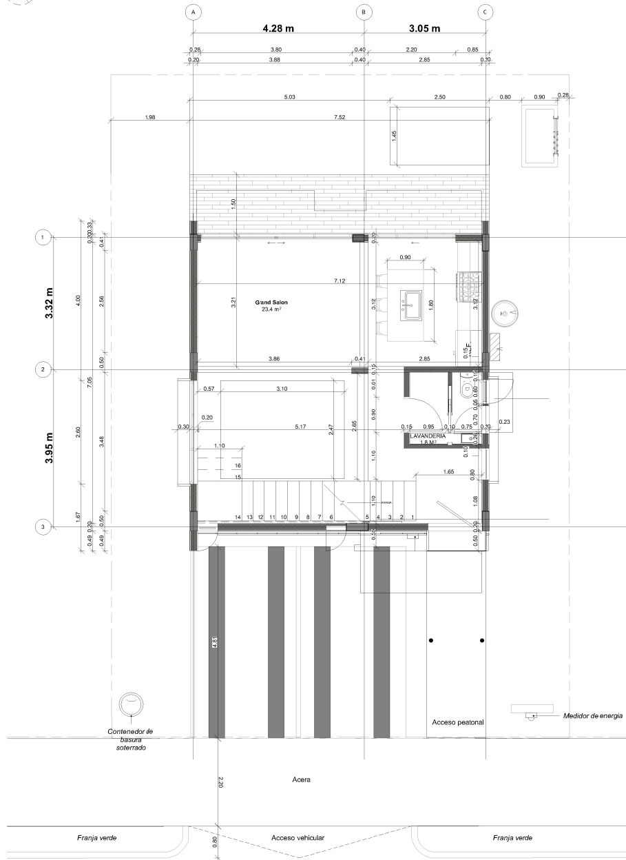
Planta dimensionada Primer Nivel
