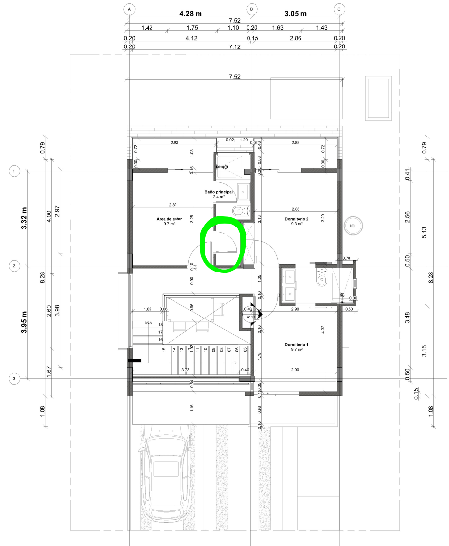
Planta dimensionada Segundo Nivel
