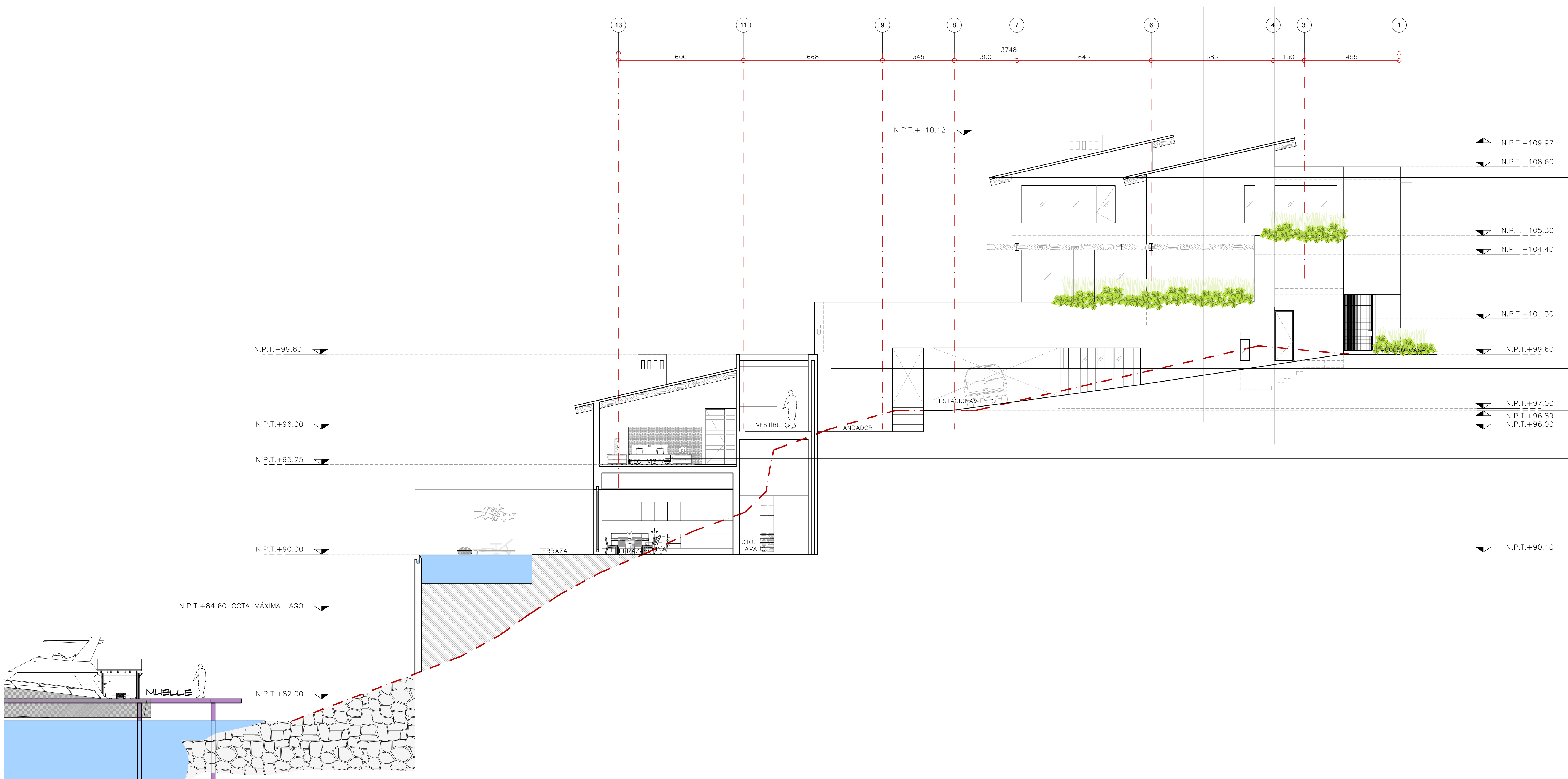
FACHADA OESTE CASA 1
