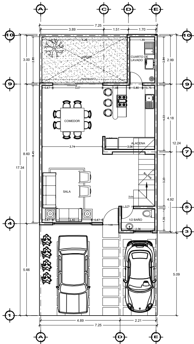
PLANTA BAJA 70.14 m 2
