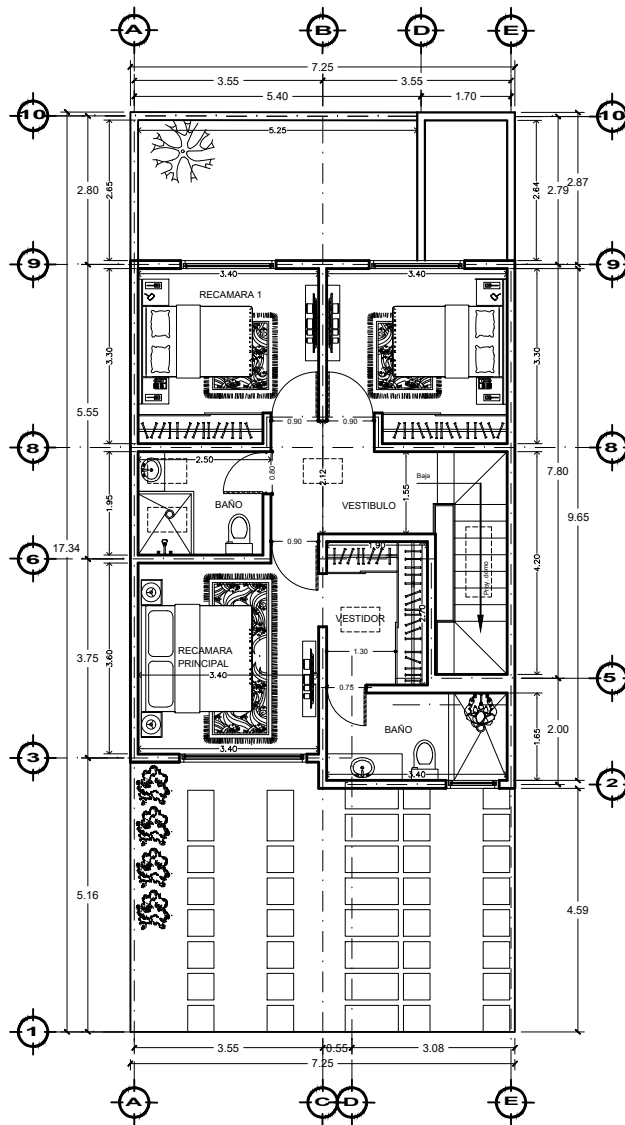
PLANTA ALTA 70.37 m 2
