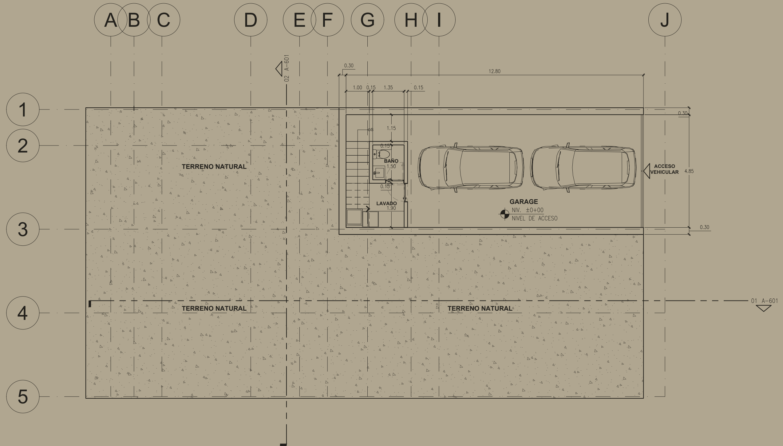
CASA TIPO 2: 5 RECAMARAS_NIVEL DE ACCESO
