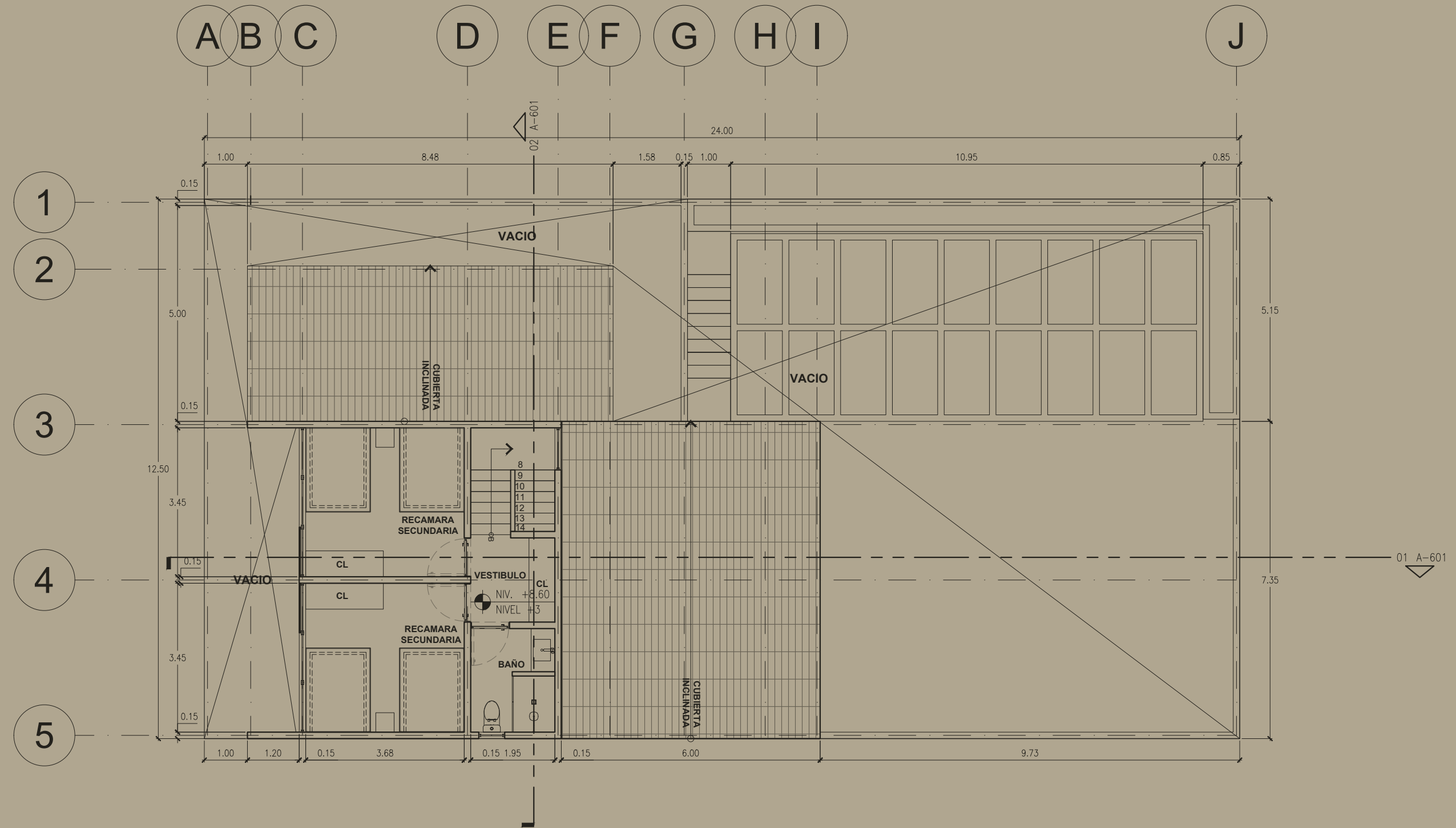
CASA TIPO 2_NIVEL +3
