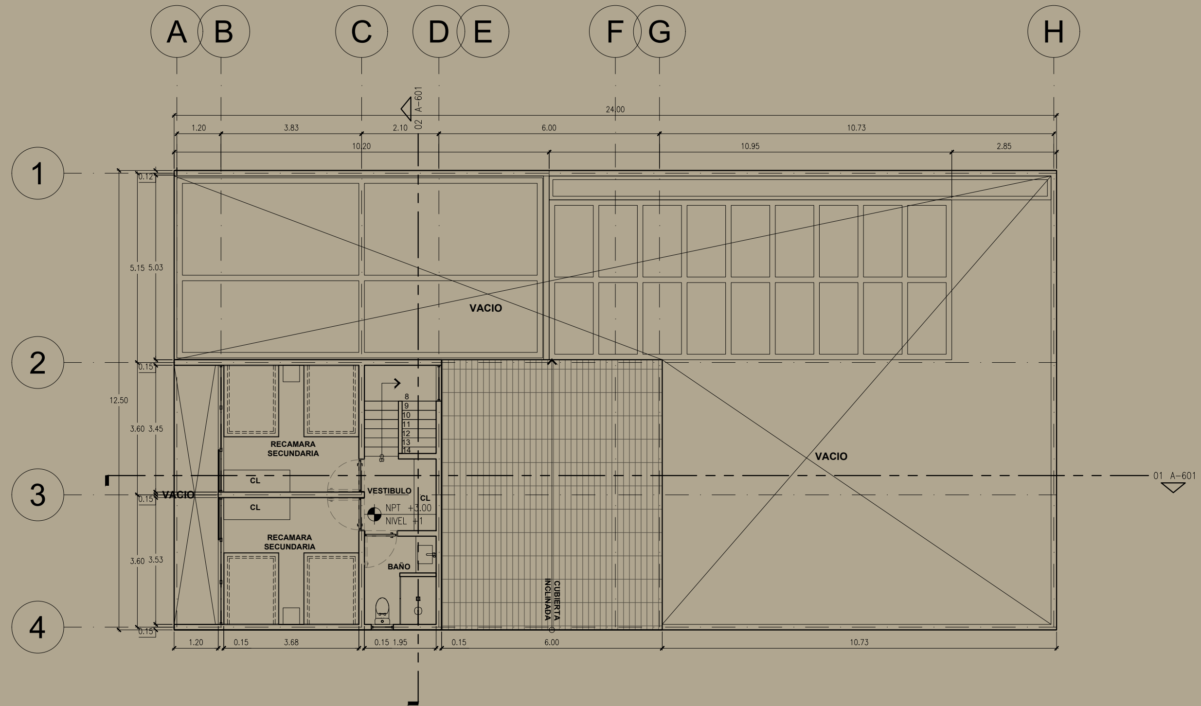
CASA TIPO 1: 4 RECAMARAS_NIVEL +1
