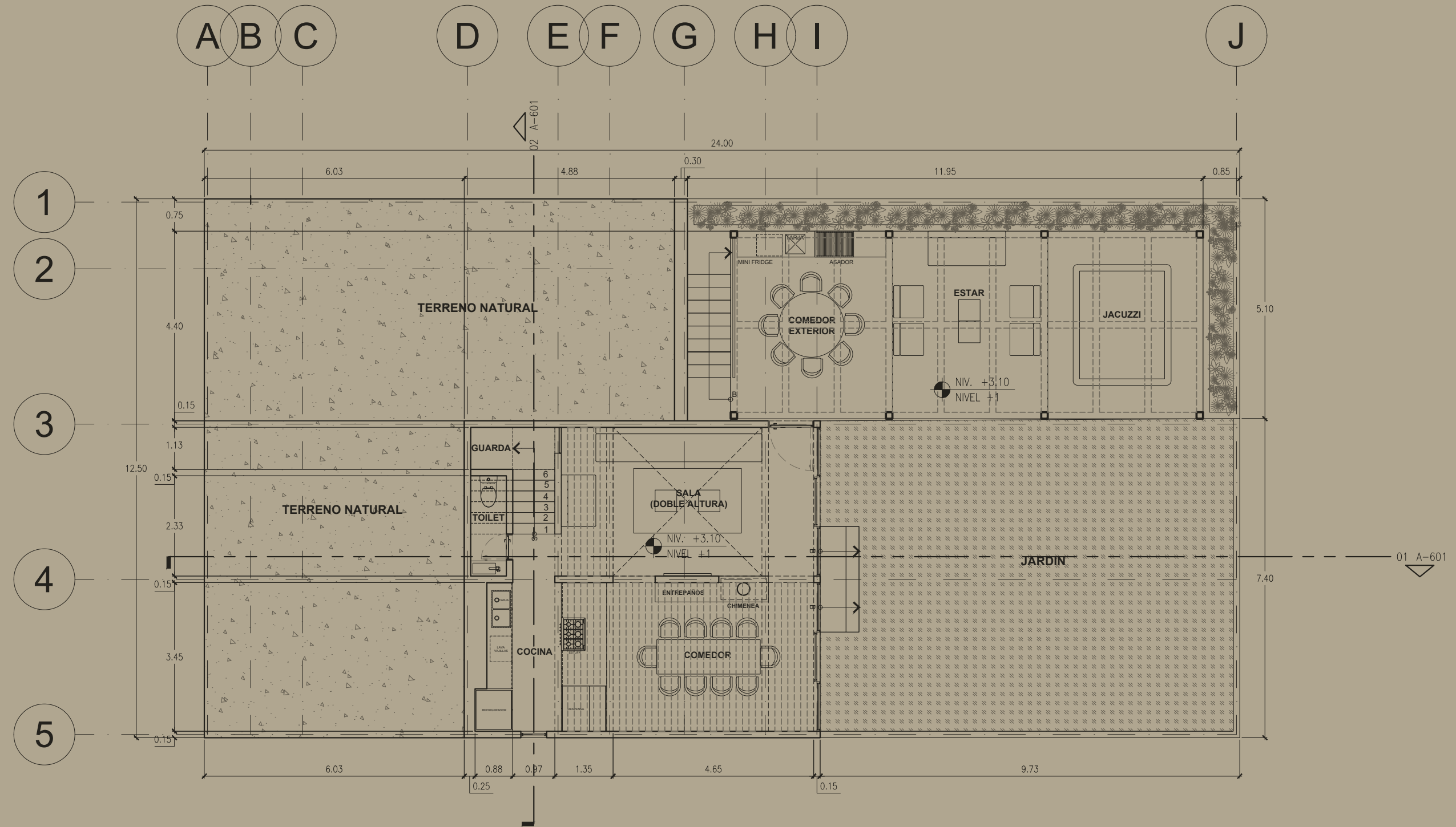
CASA TIPO 2: 5 RECAMARAS_NIVEL +1
