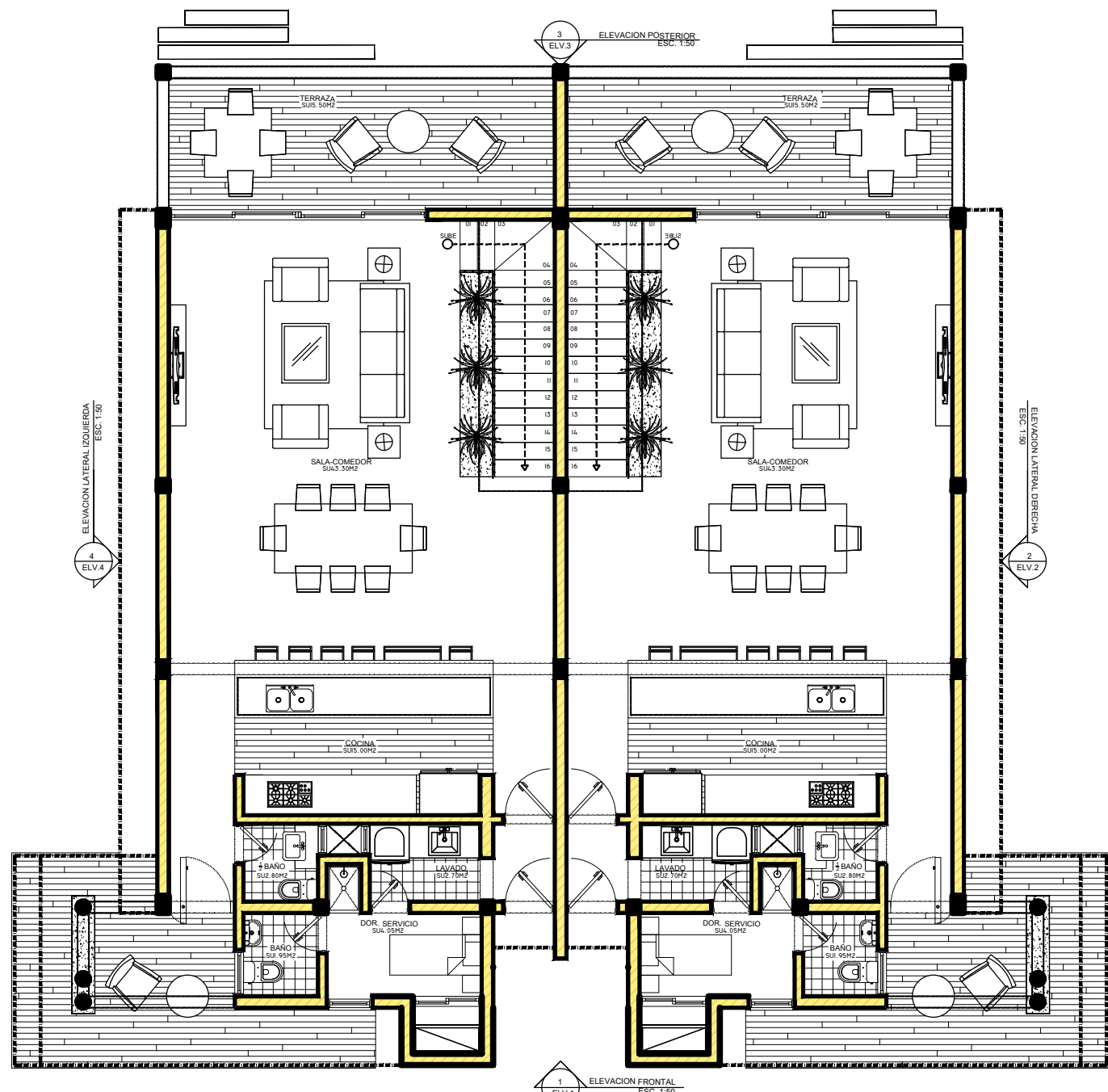
ARQ.#1 NIVEL.2 PLANTA ARQUITECTONICA 1ER NIVEL A LA 2- NIVEL ESC. 1:50
