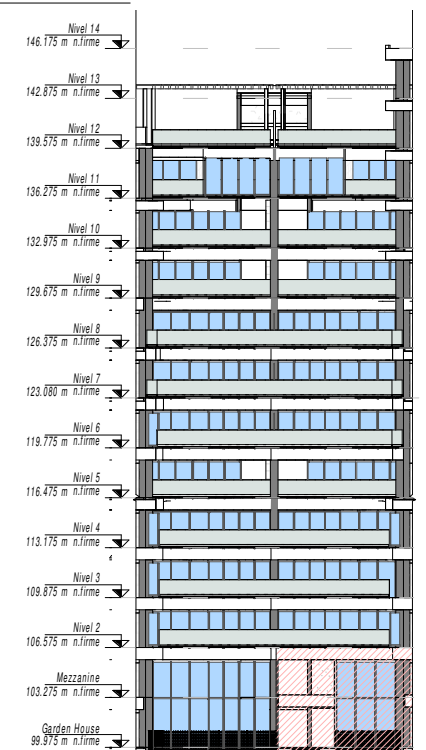
4 Ubicación en Torre (Fachada) Escala 1:500
