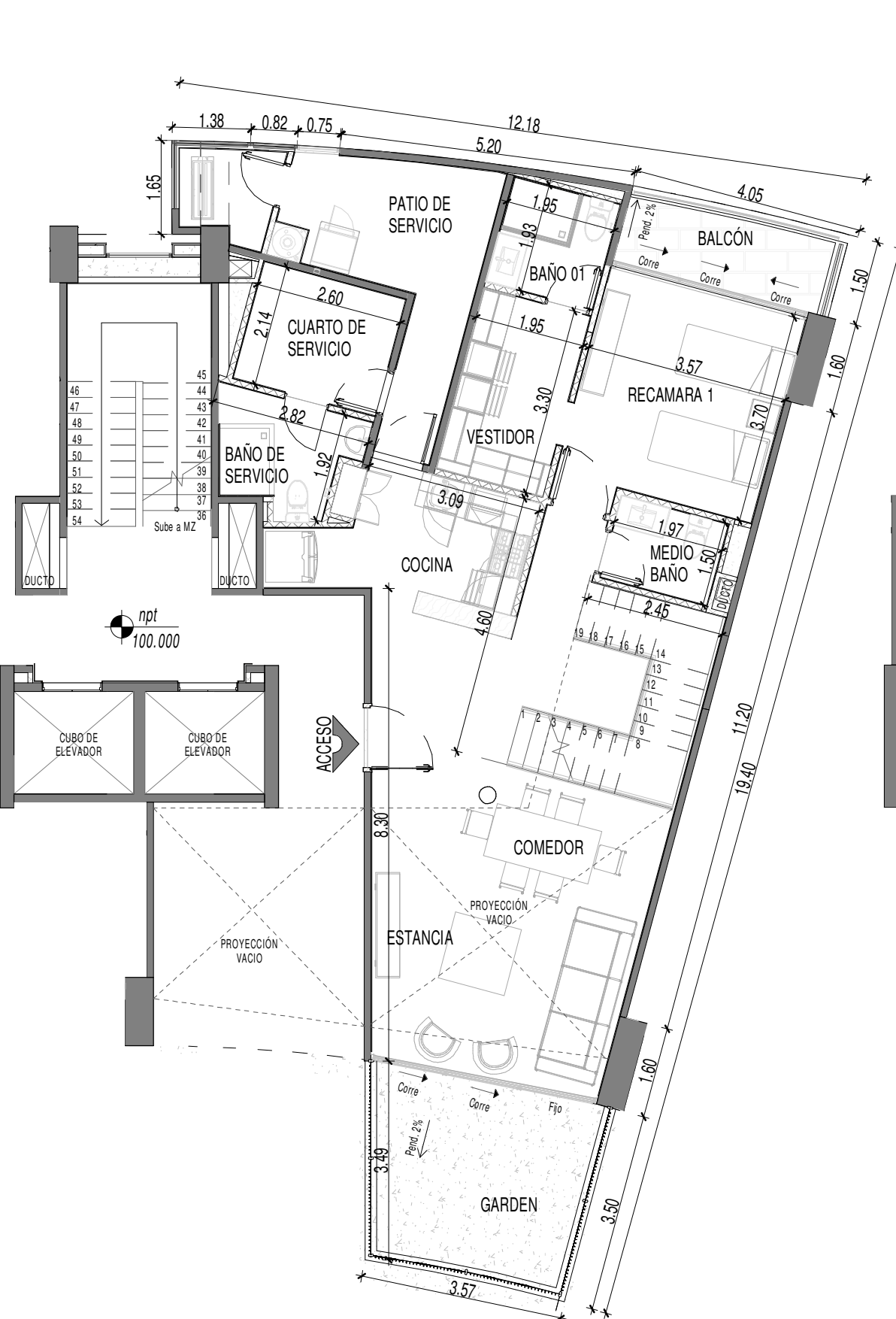
1 Arquitectónico Amueblado Garden House Escala 1:100
