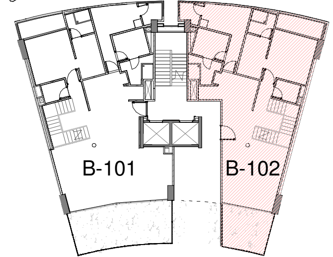
3 Ubicación en Torre Escala 1:300
