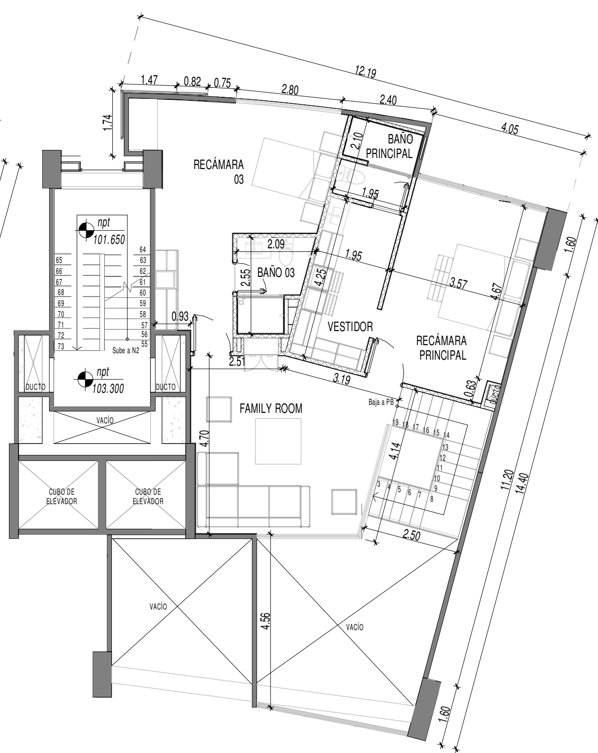
3 Ubicación en Torre Escala 1:300
