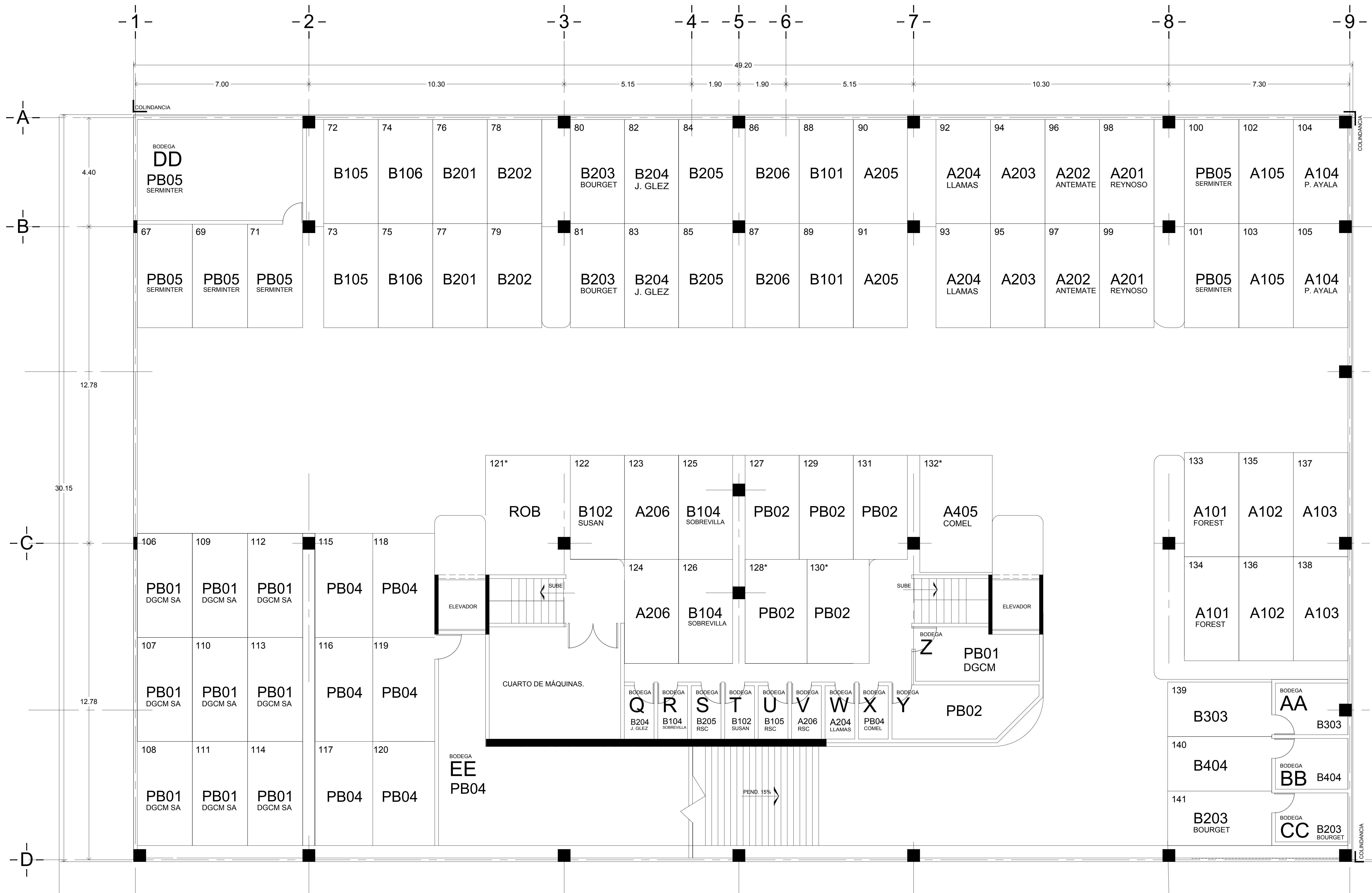
PLANTA SÓTANO 2
