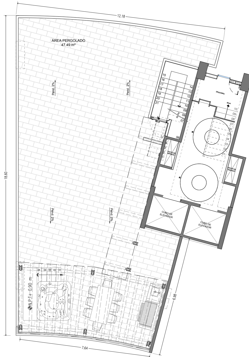
ARQUITECTÓNICO AMUEBLADO ROOFTOP
