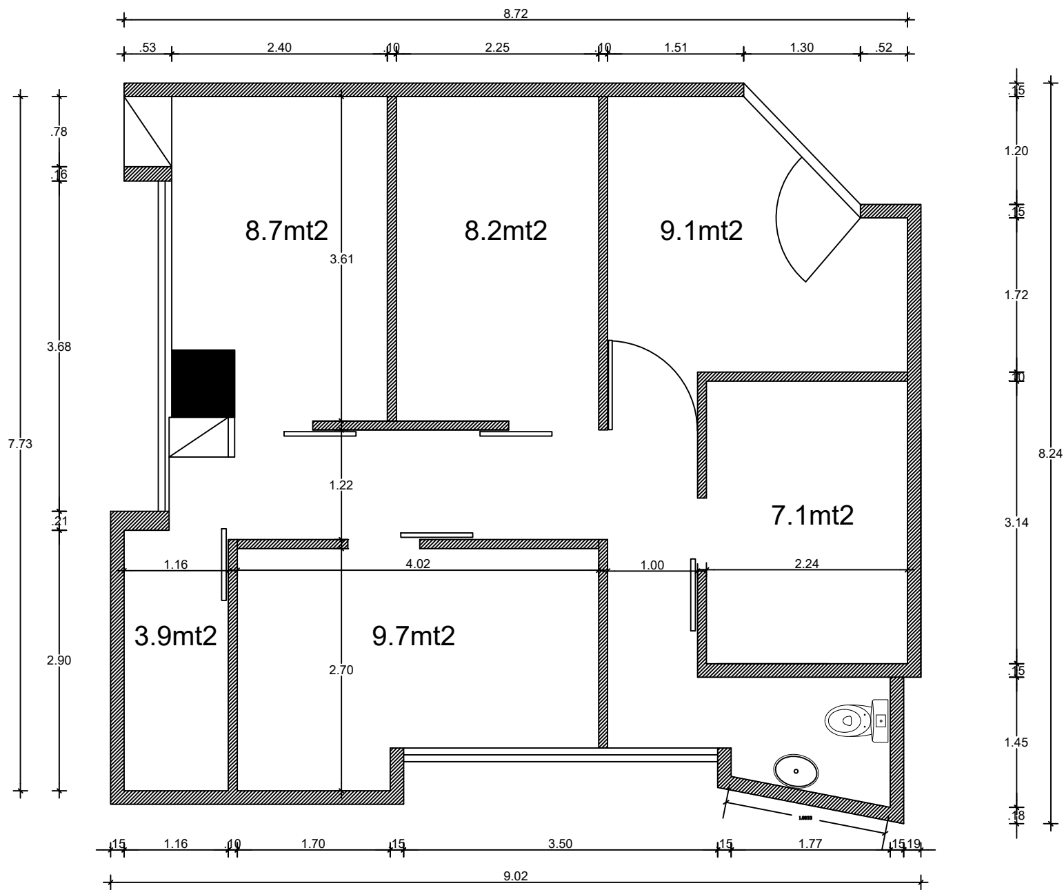
PLANTA DIMENSIONADA
