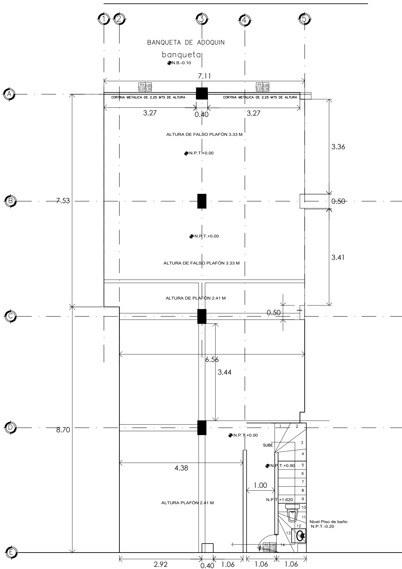
planta baja
