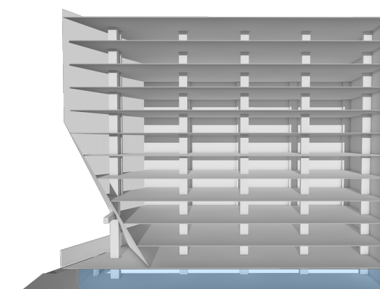
CORTE ESQUEMÁTICO
