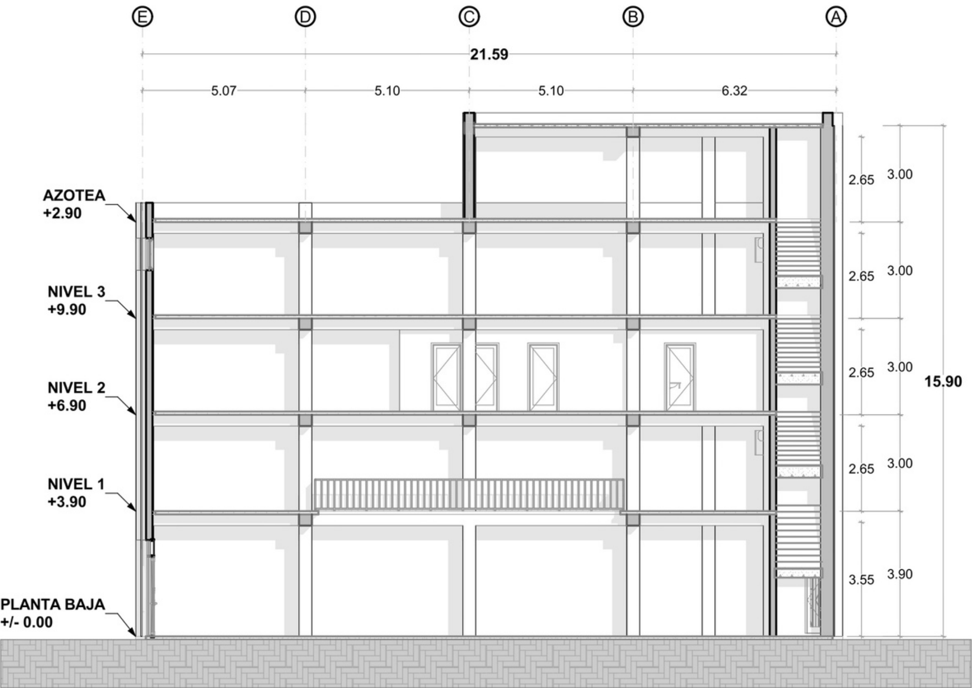
CORTE LONGITUDINAL
