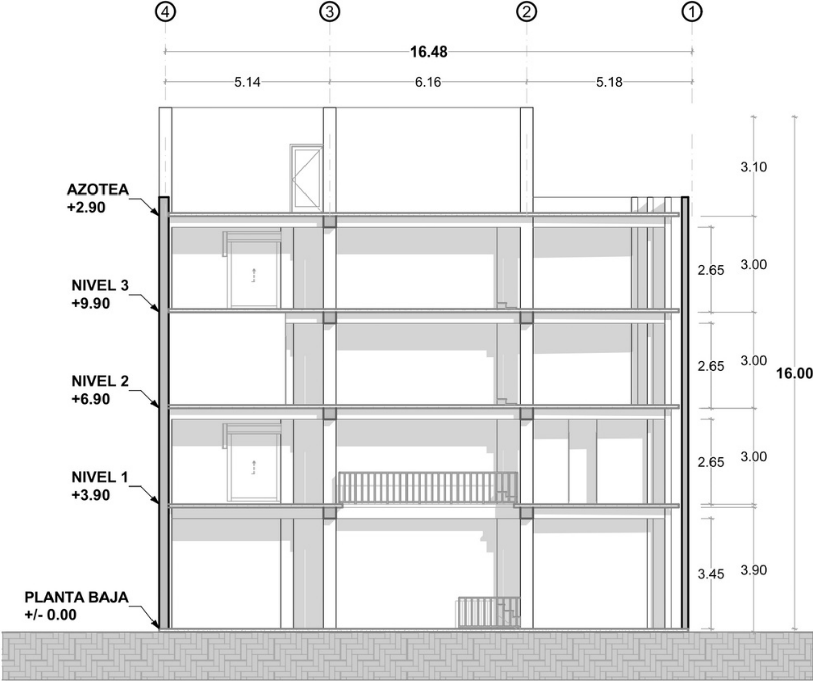
CORTE TRANSVERSAL
