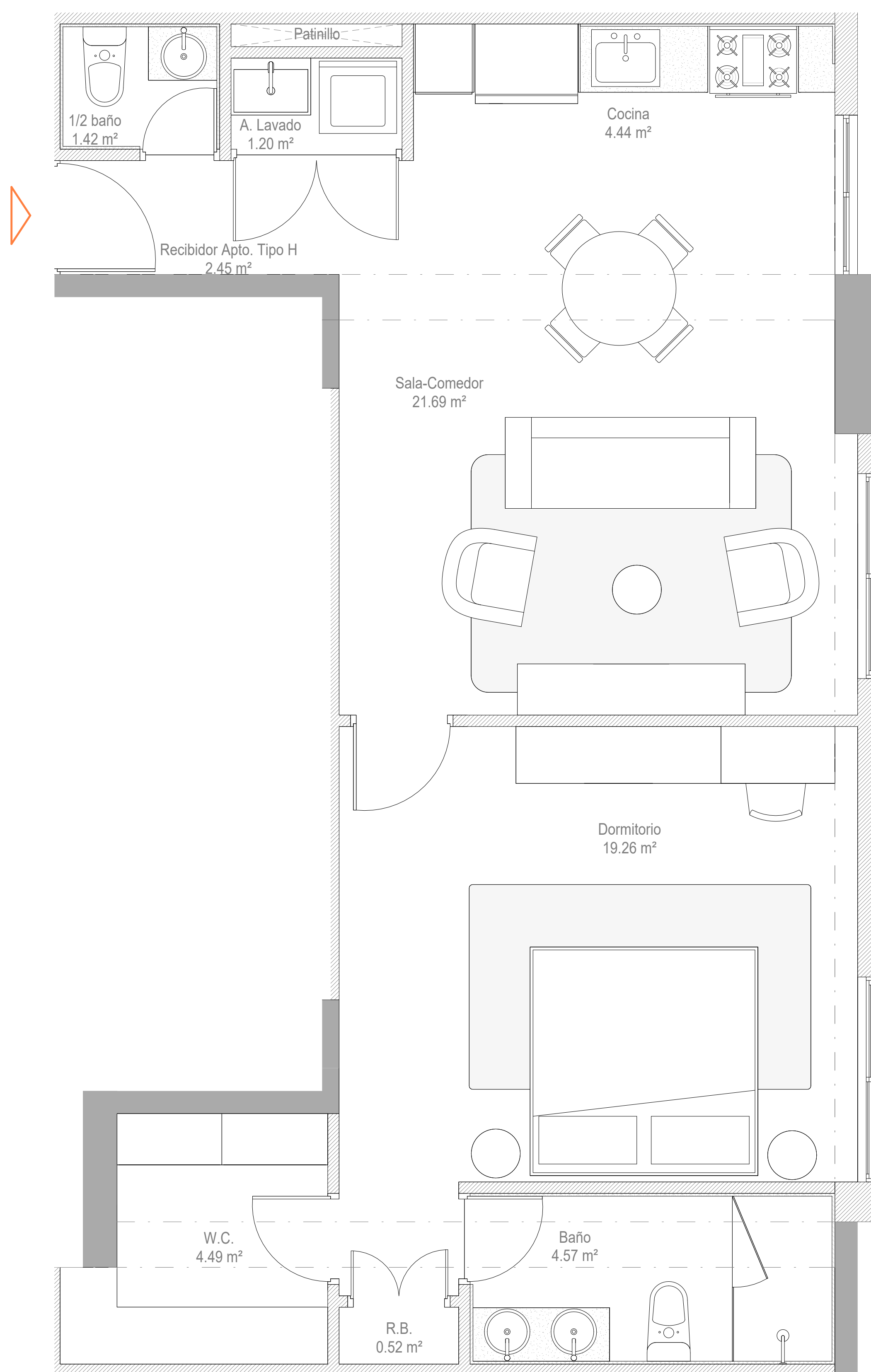
2 PLANTA ARQ. AMUEBLADA APTOS. TIPO H A04 / 1:25
