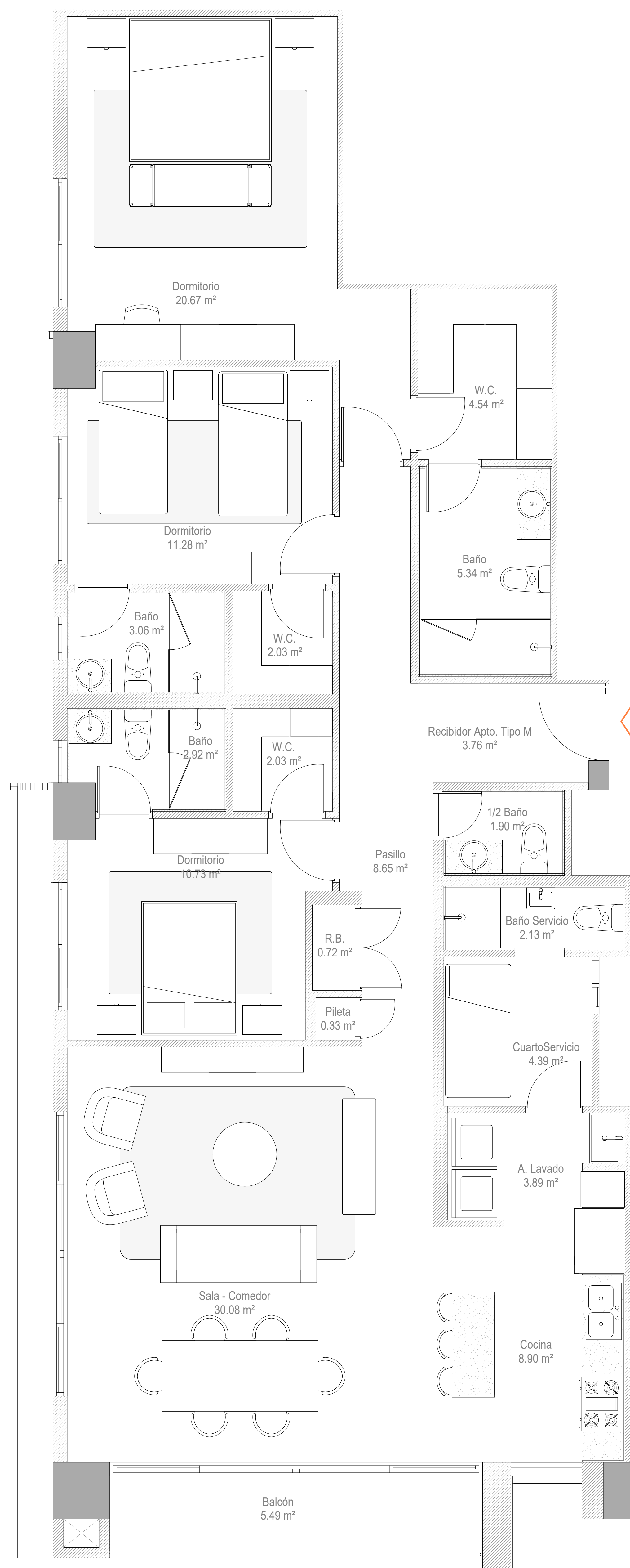
2 PLANTA ARQ. AMUEBLADA NIVEL 11 A13 1:30
