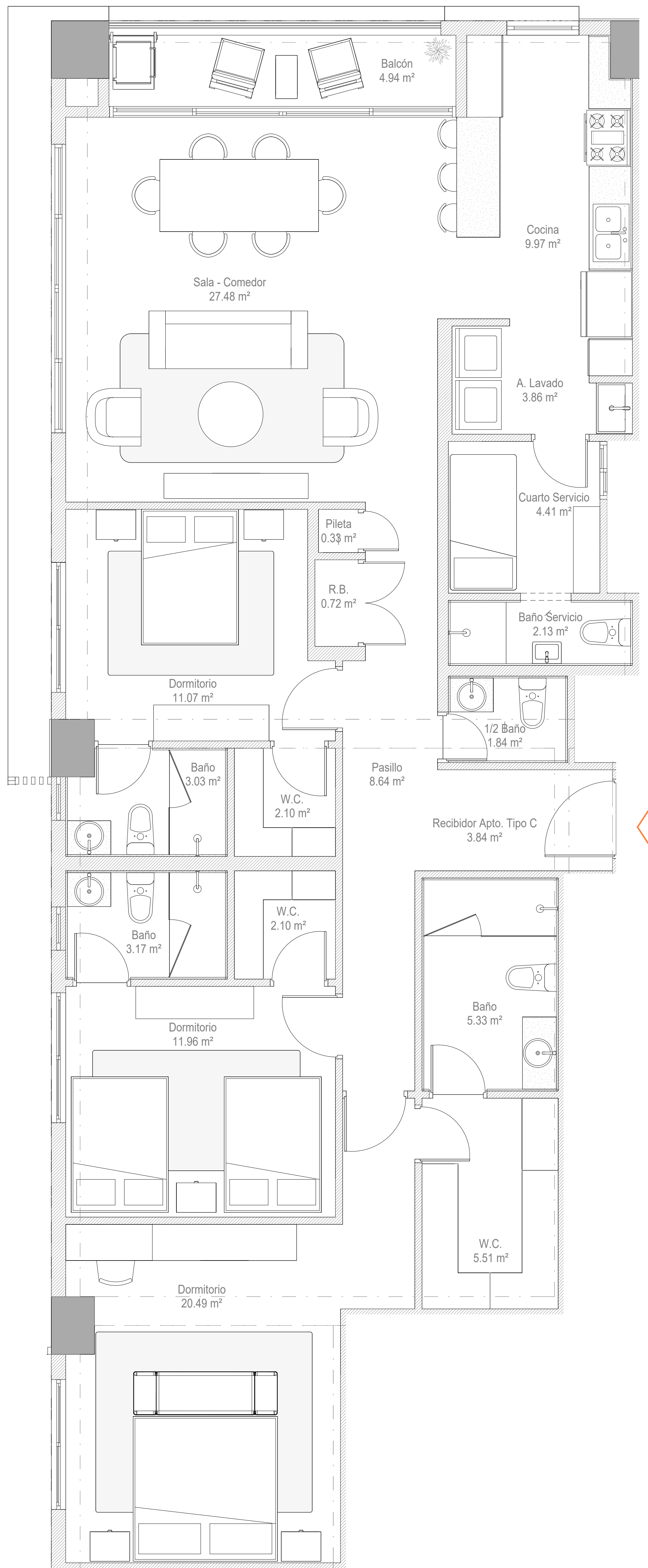
2 PLANTA ARQ. AMUEBLADA APTO. TIPO C A11 1:30
