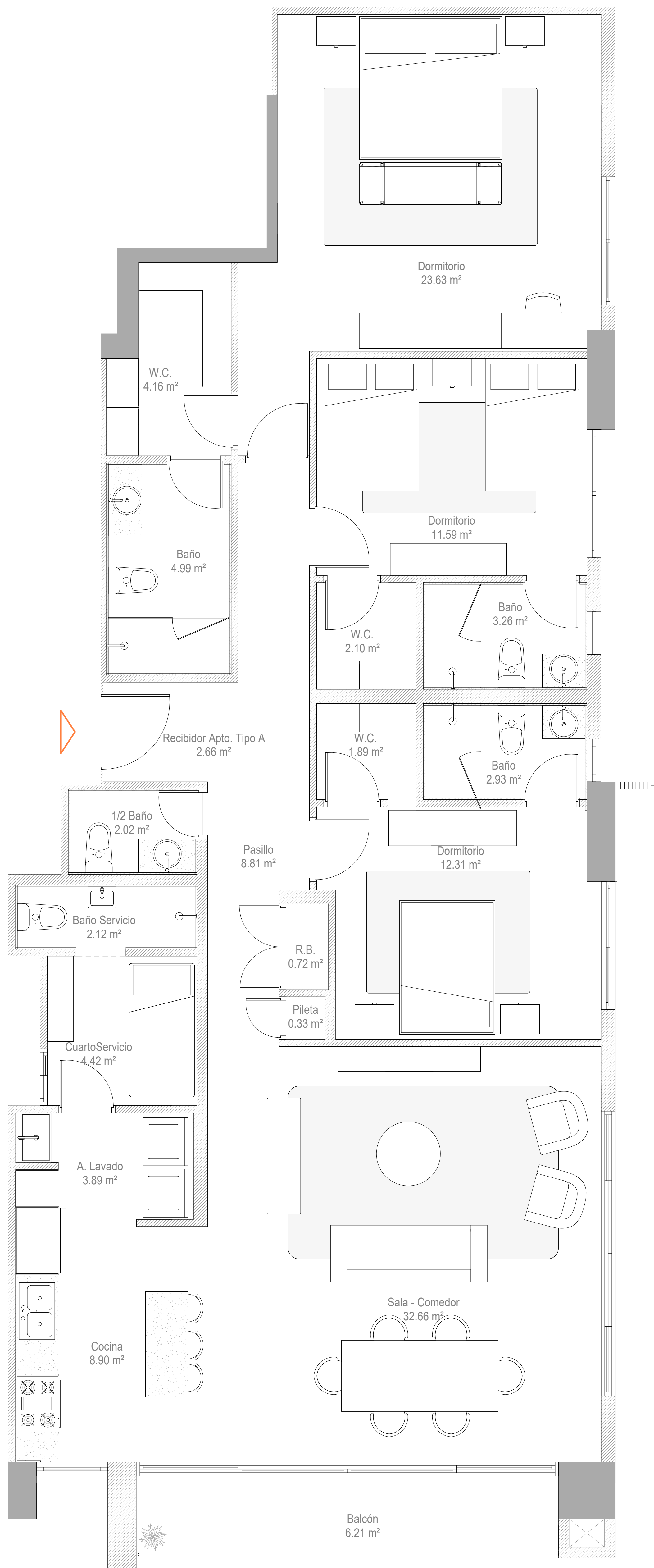
1 PLANTA ARG. AMUEBLADA NIVEL 11 AT4 / 1:30
