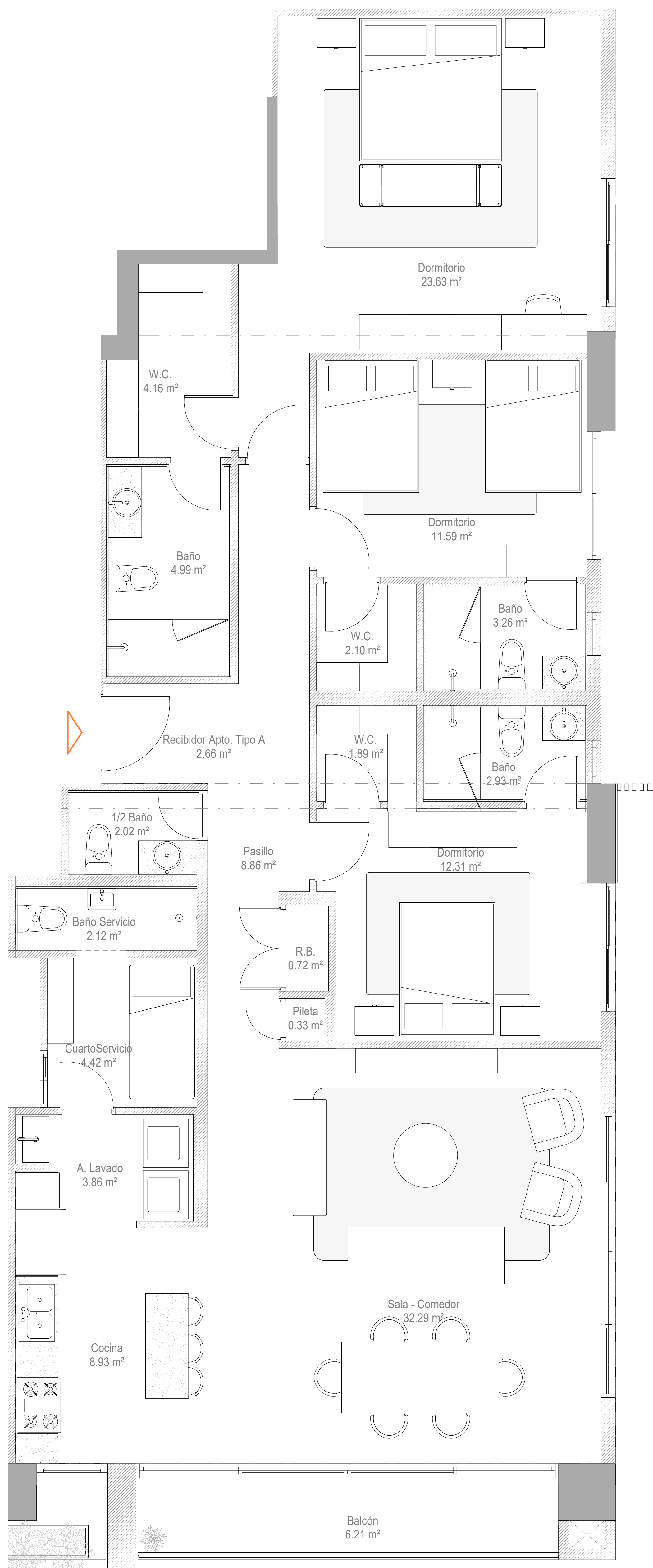
2 PLANTA ARQ. AMUEBLADA APTO. TIPO A 110/1-30
